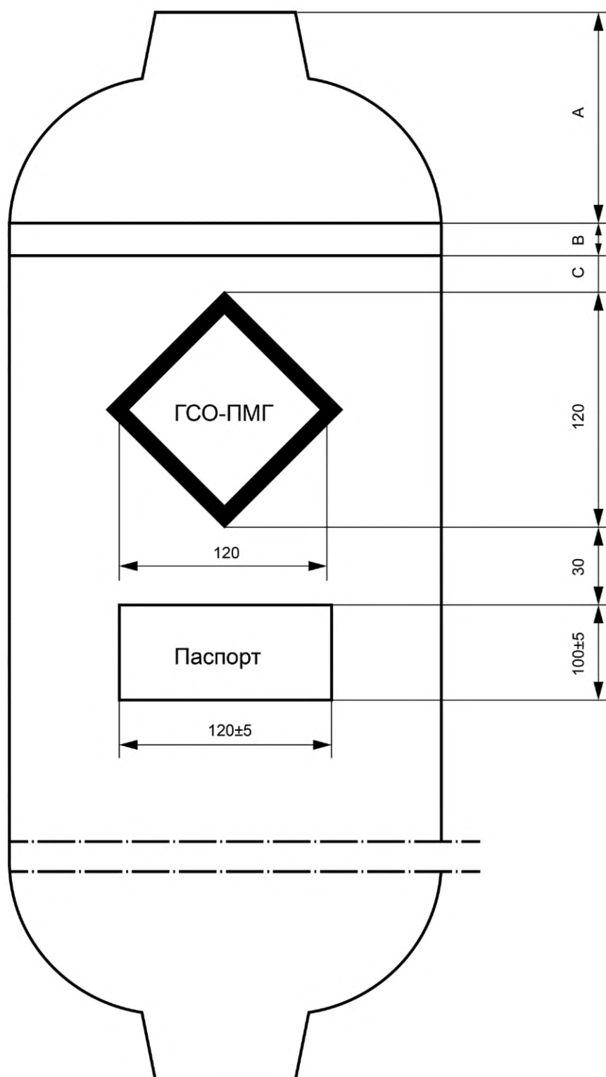
Рисунок В.1 — Маркировка баллона
