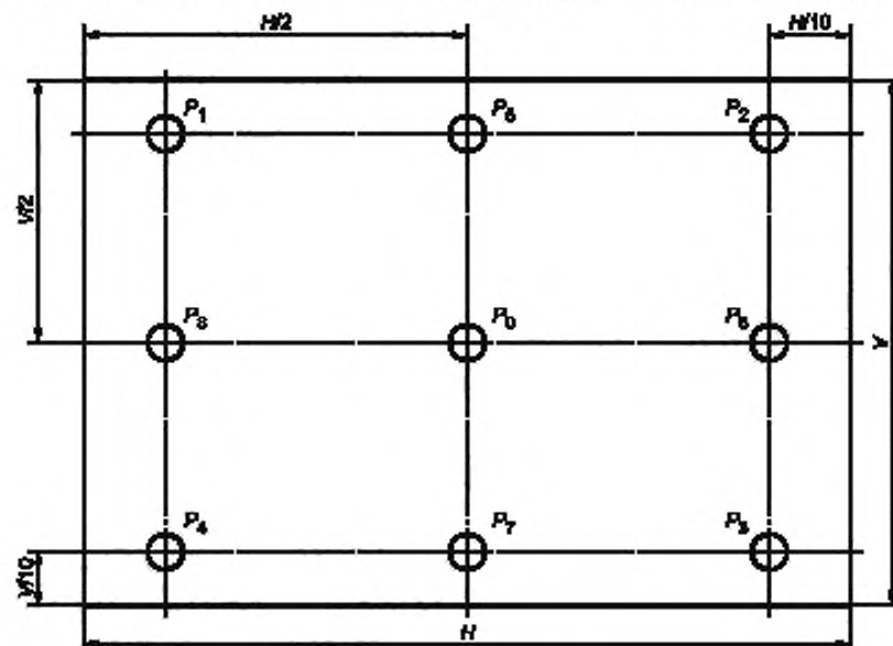
Рисунок 3 — Точки измерения
