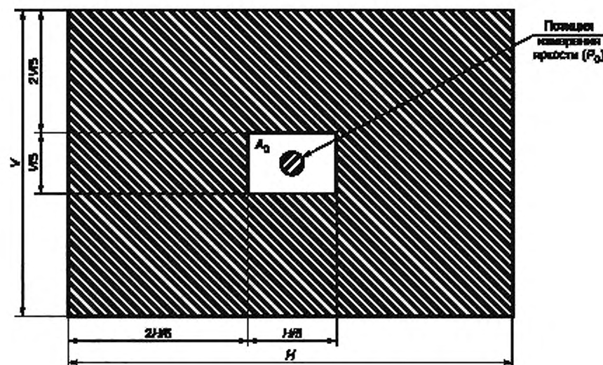
Шаблон для измерения яркости 4 % окна
