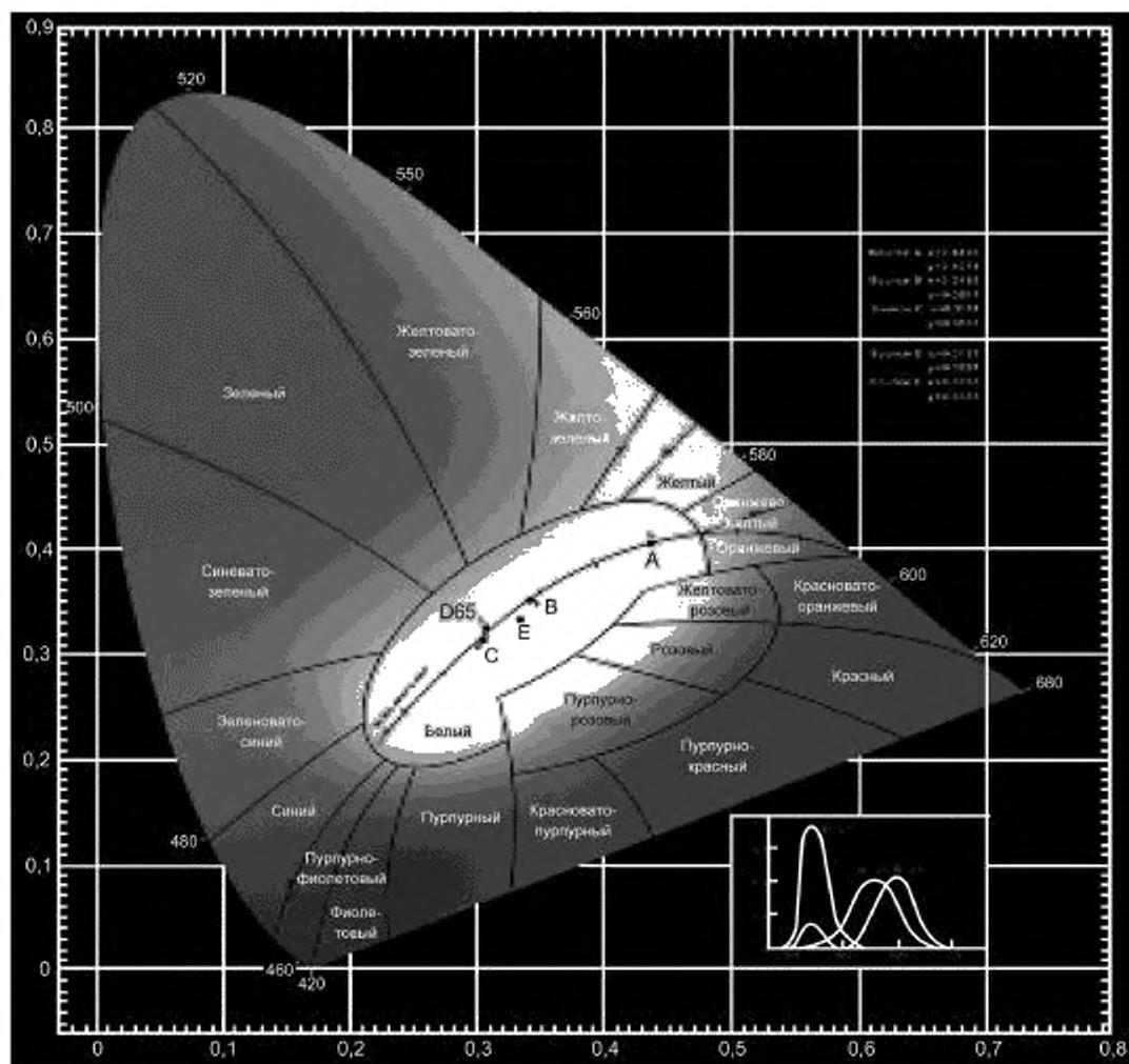
Рисунок D.1 — График цветности XYZ CIE 1931
