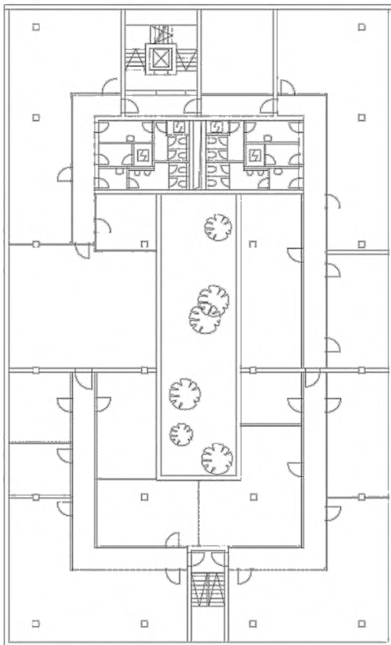
Рисунок 5 — План этажа
