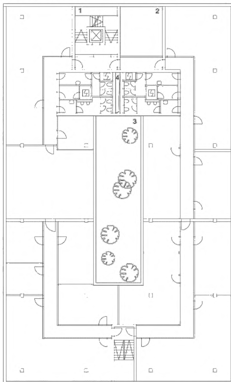
Рисунок 6 — Нефункциональная зона этажа
