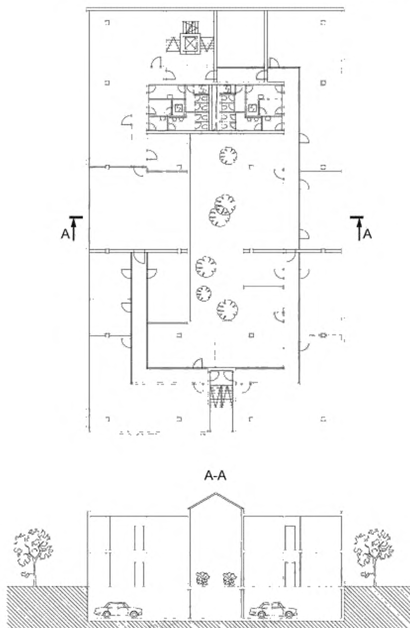
Рисунок 4 — Постлабный план здания и план верхнего этажа
