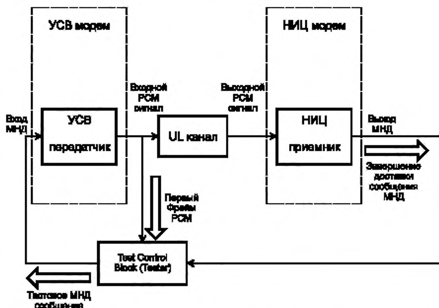
Рисунок Е.2 — Общая схема проведения тестирования для определения среднего времени передачи сообщения МНД для различных вариантов голосового кода AMR и GSM-FR
