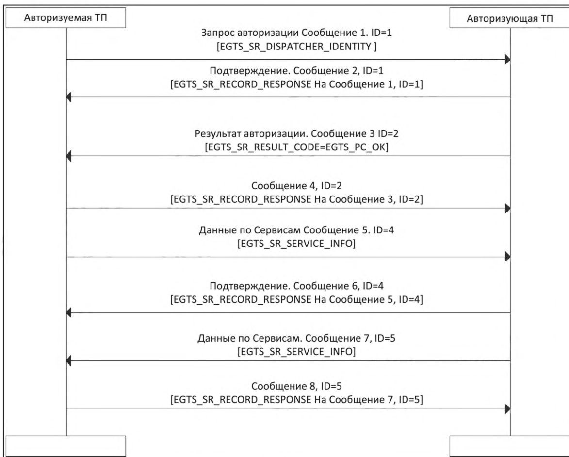
Рисунок В.7 — Алгоритм обмена сообщениями на этапе авторизации авторизуемой ТП на авторизирующей ТП
