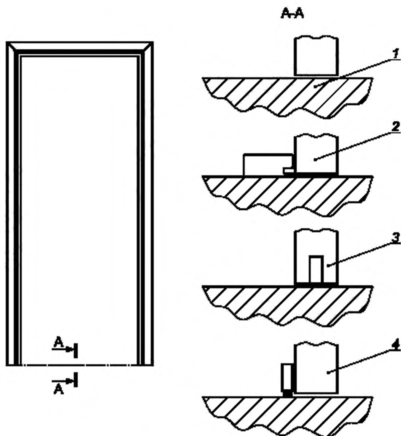
1 — без порога; 2 — с приставным порогом; 3 — с выдвижным порогом встроеного типа; 4 — с выдвижным порогом накладного типа
