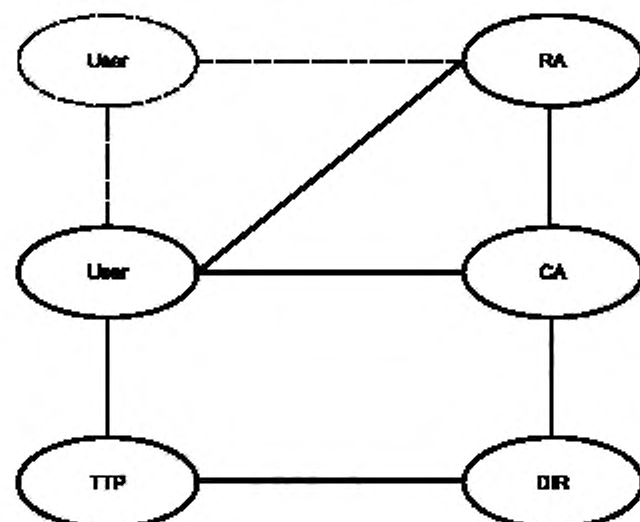
Рисунок D.1 — Модель управления ключами
