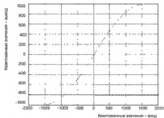
Рисунок J.2 — Передаточная функция усилителя
