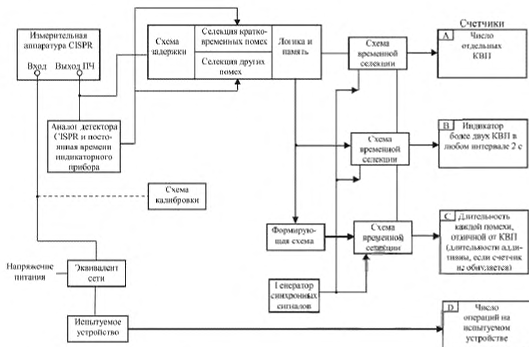
Рисунок 12 — Пример анализатора помех
