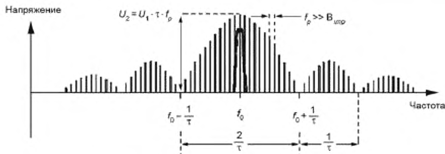
Рисунок Е.5 — Фильтрация, когда B_{\text{шпр}} намного меньше частоты повторения импульсов
