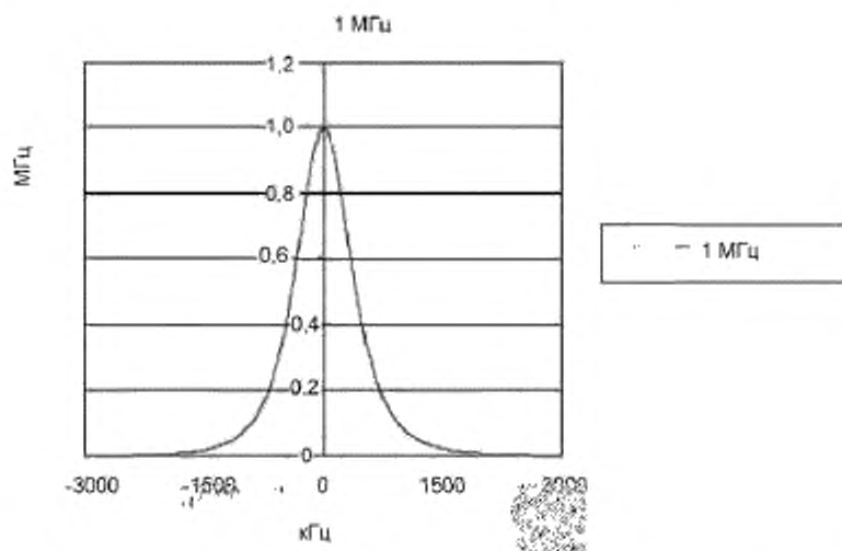
Рисунок Е.8 — Пример нормализованной линейной функции избирательности
