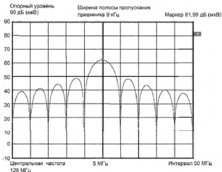
Рисунок Е.3 — Спектрограмма импульсно-модулированного сигнала при ширине импульсов 200 нс
