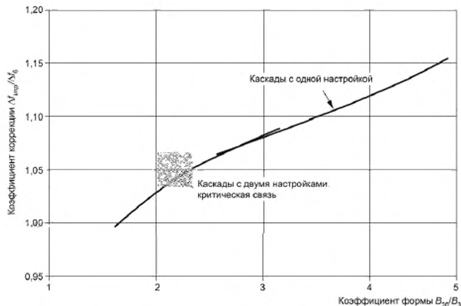
Рисунок Е.1 — Коэффициент коррекции для оценки отношения B_{mp}/B_6 для других типов настраиваемых каскадов
