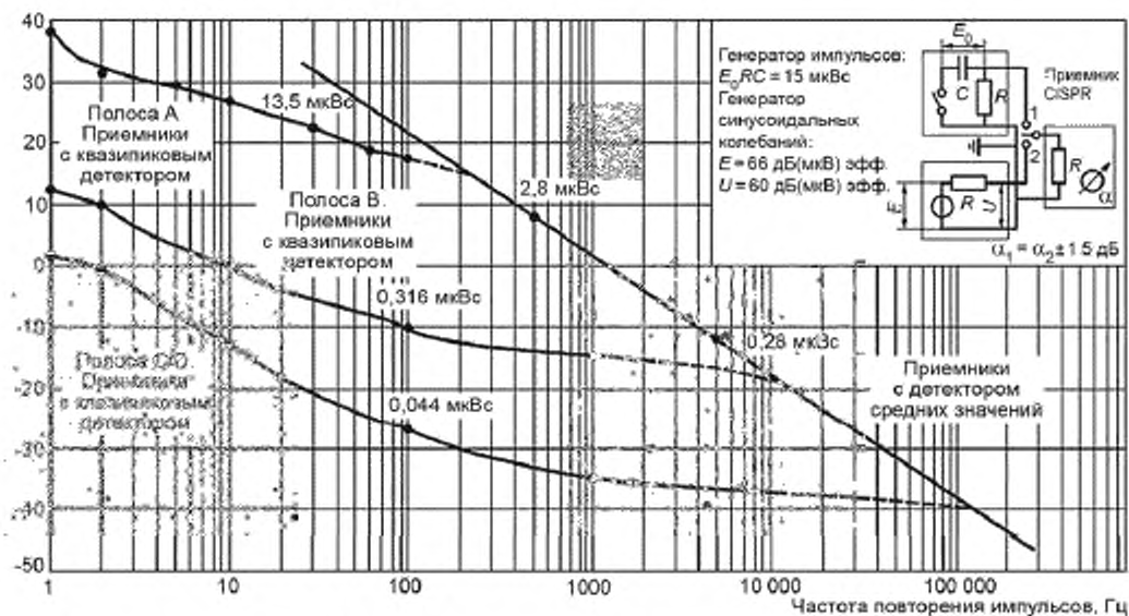
Рисунок 4 — Теоретические кривые импульсной характеристики приемников с квазипиковым детектором и детектором средних значений
