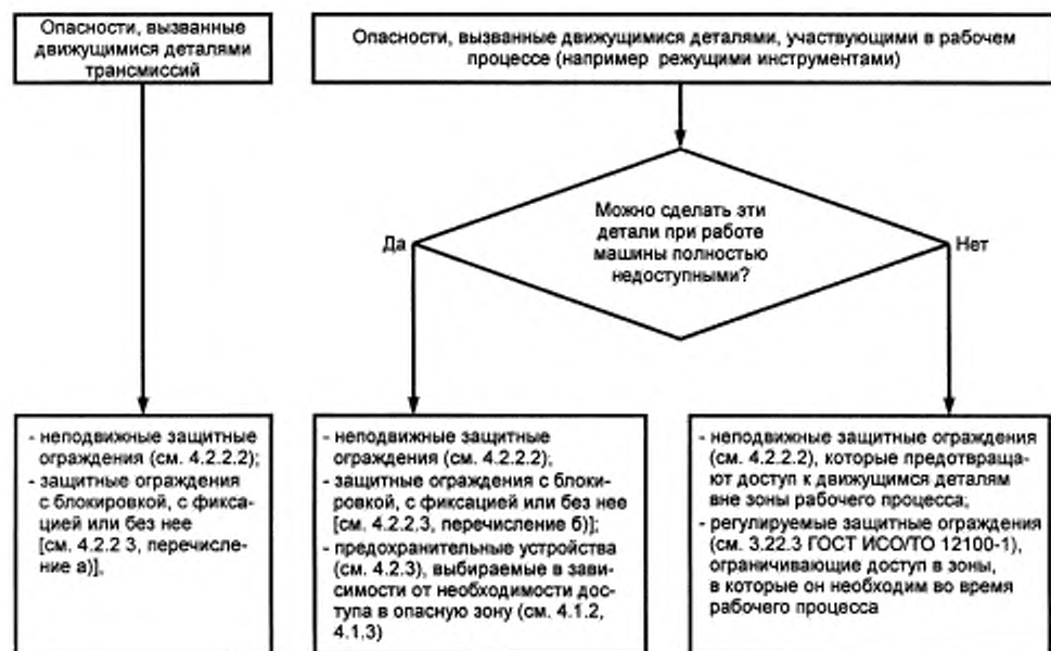
Рисунок 1 — Рекомендации для выбора защитных ограждений и предохранительных устройств при опасностях, связанных с движущимися деталями
