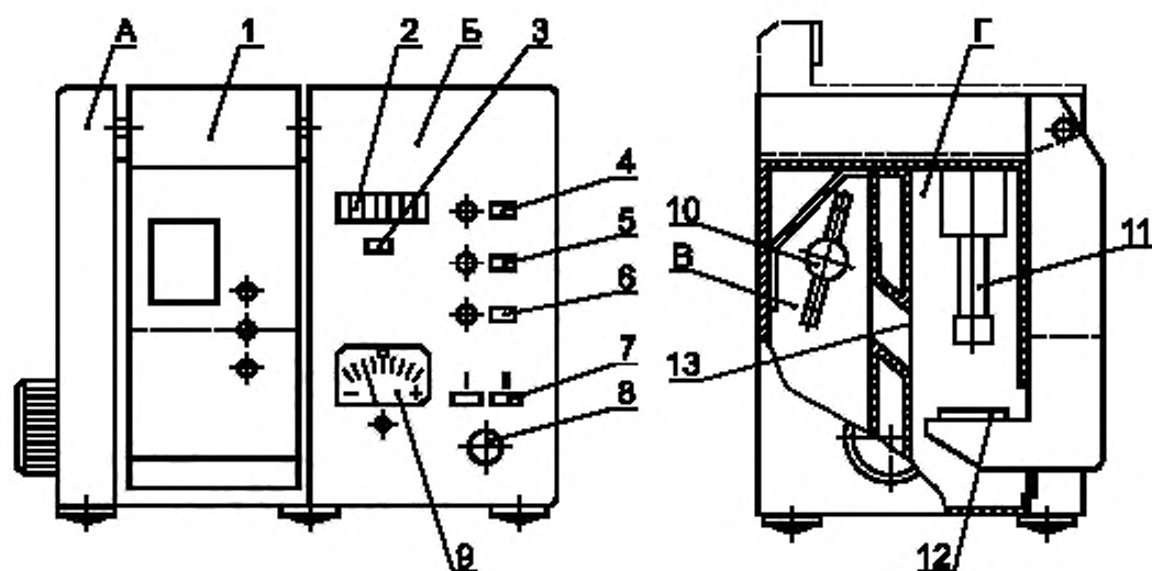
А — блок индикации; Б — электронный блок управления; В — отсек излучателя; Г — испытательный отсек; 1 — кювета; 2 — счетчик времени; 3 — кнопка сброса счетчика времени; 4 — кнопка выключения прибора; 5 — кнопка выключения ртутной лампы; 6 — кнопка выключения ФЭУ; 7 — кнопка переключения режимов; 8 — индикатор напряжения; 9 — регулятор порога чувствительности; 10 — ртутная лампа ДРК 120; 11 — фотоэлектронный умножитель; 12 — кассета с образцом; 13 — светофильтр УФС-8
