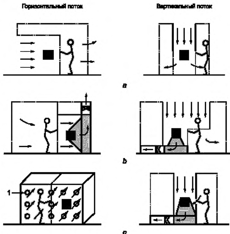
a — защита продукта; b — защита персонала и окружающей среды; c — защита персонала, продукта и окружающей среды; I — направление потока перпендикулярно к плоскости рисунка
