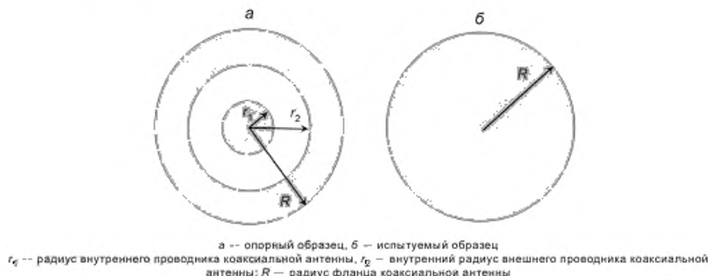
Рисунок 9 — Размеры образцов материала
