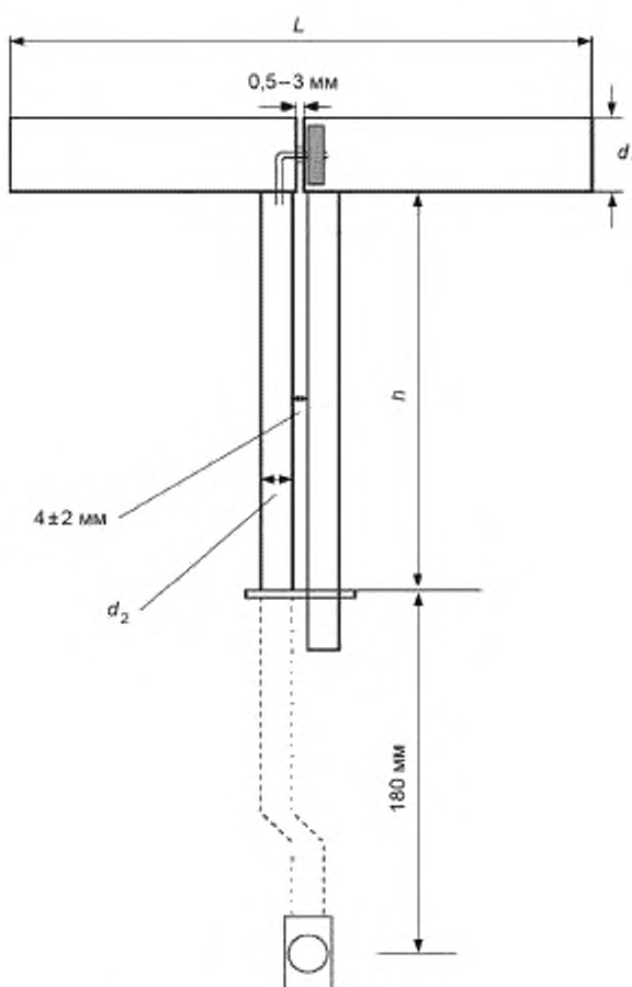
Рисунок 1 — Размеры полуволнового диполя
