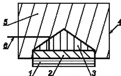
1 — пьезопластинка; 2 — контактный слой; 3 — механический демпфер; 4 — металлический экран; 5 — компаунд; 6 — высокочастотный кабель
