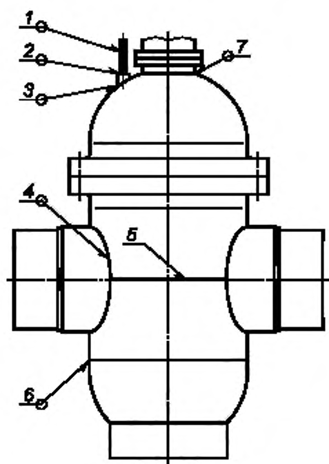
1 — 7 — сварные швы
