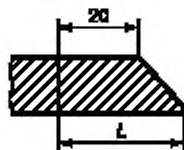
Рисунок 7 — Присоединительный конец под приварку
