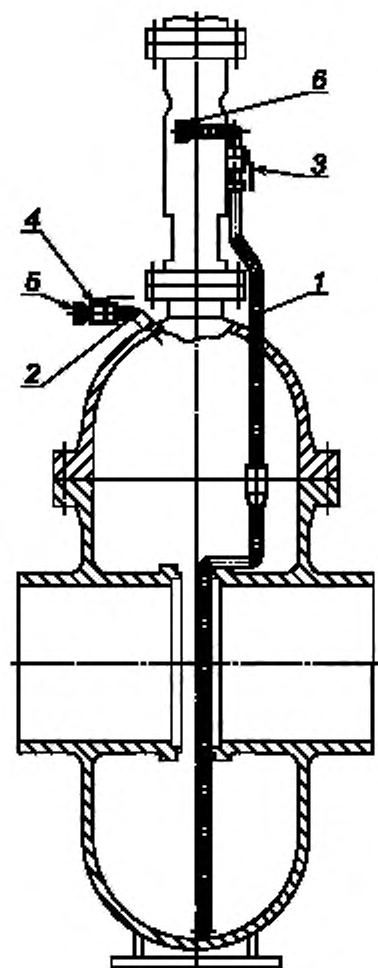
1 — дренажный трубопровод; 2 — спускной трубопровод; 3, 4 — запорная арматура, 5, 6 — заглушка
