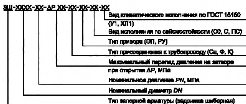
Рисунок 1 — Схема условного обозначения задвижки
