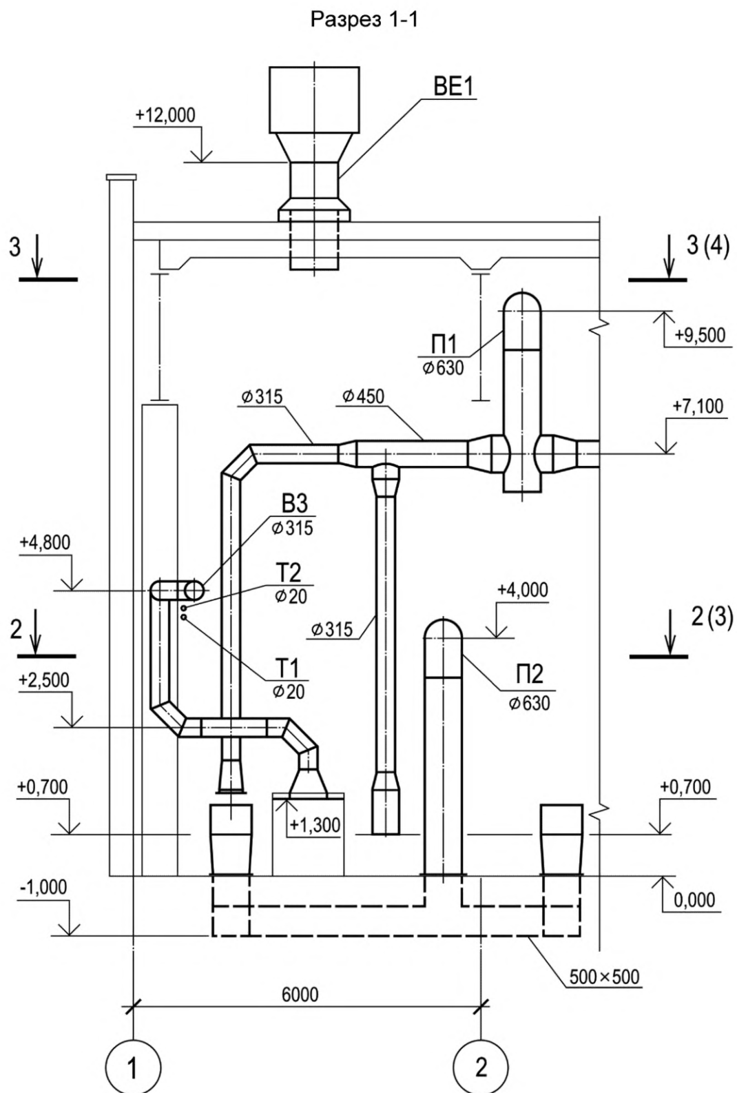
Рисунок Б.3 — Пример выполнения разреза систем
