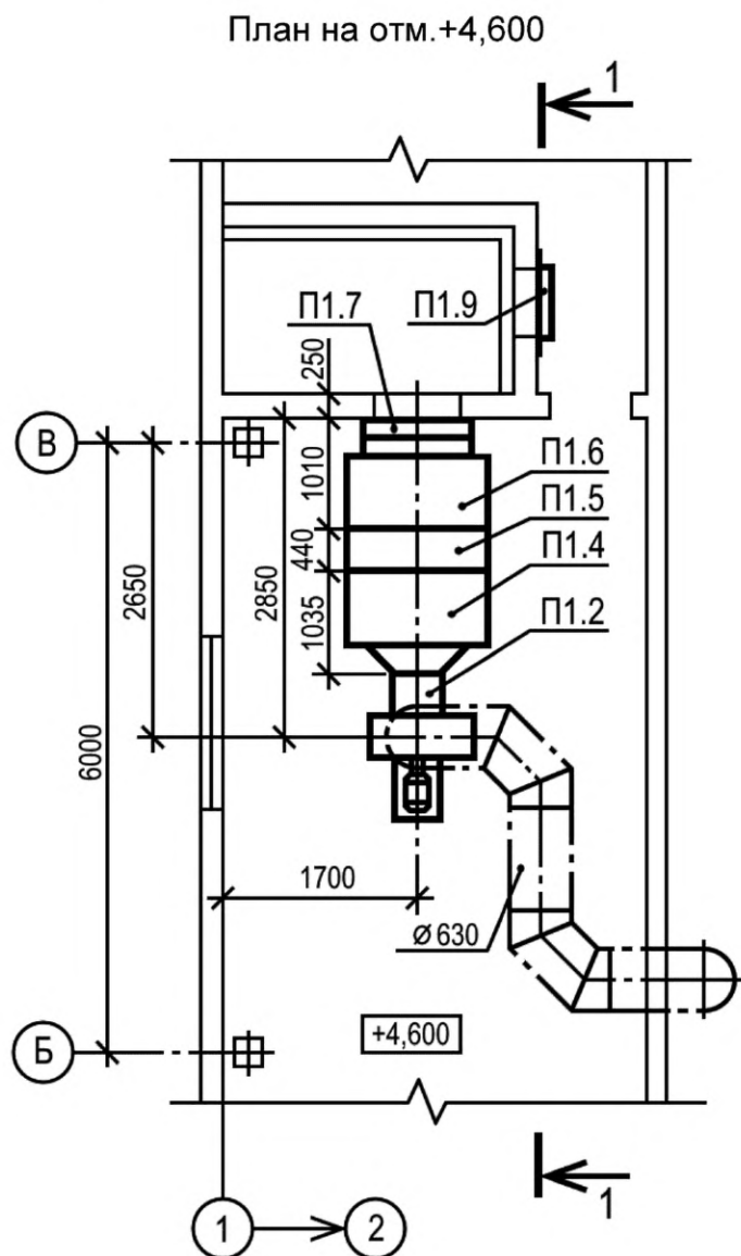
Рисунок Д.1 — Пример выполнения плана установки
