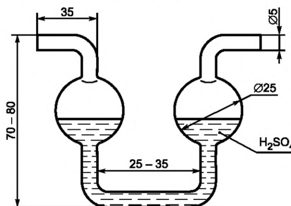
Рисунок 2 — Насадка
