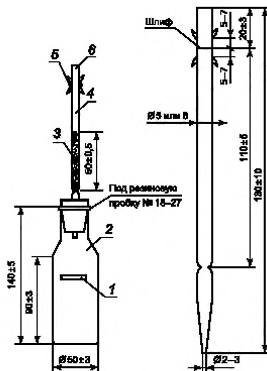
1 — метка, соответствующая объему 0 см 3 ; 2 — склянка; 3 — ватный тампон; 4 — длинная стеклянная трубка (перетяжка в трубке необязательна); 5 — бромно-ртутная бумага; 6 — короткая стеклянная трубка (перетяжка в трубке необязательна)
