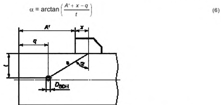
Рисунок 6 — Определение угла ввода с использованием бокового отверстия в настроечном образце
