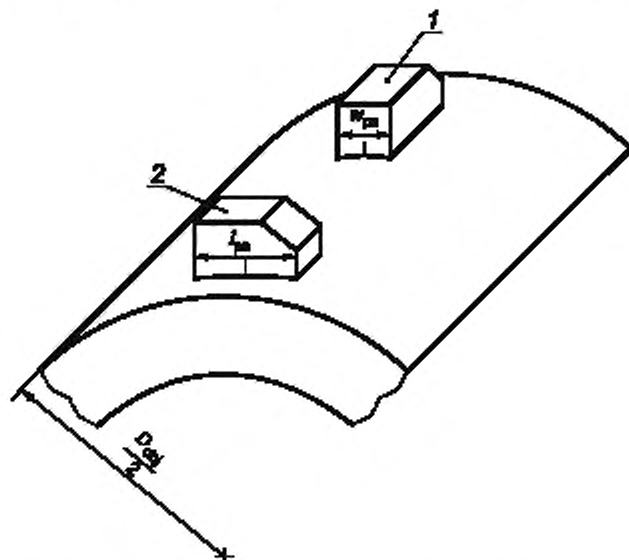
Рисунок 1 — Длина l_{ps} и ширина w_{ps} контактной поверхности преобразователя в направлении кривизны объекта контроля
