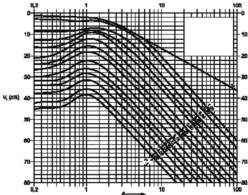
Рисунок 10 — Общая DGS-диаграмма
