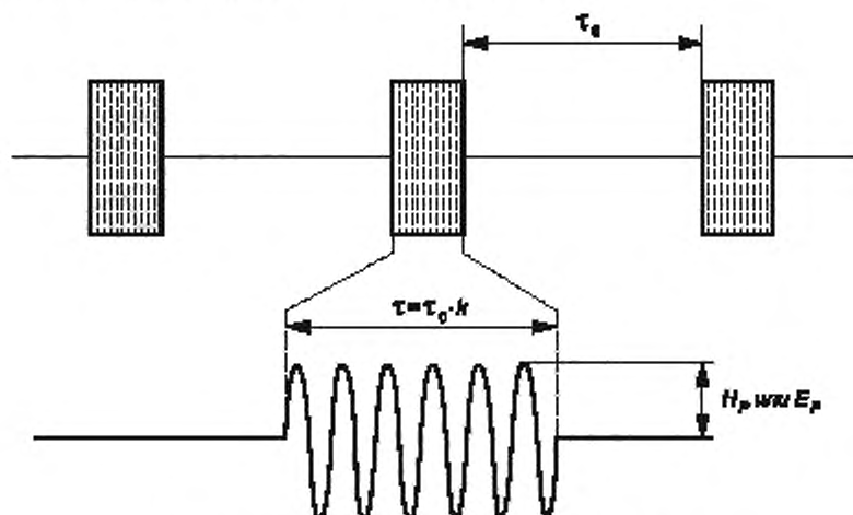
Рисунок 107 — Сигнал помехи на частотах выше 1 кГц
