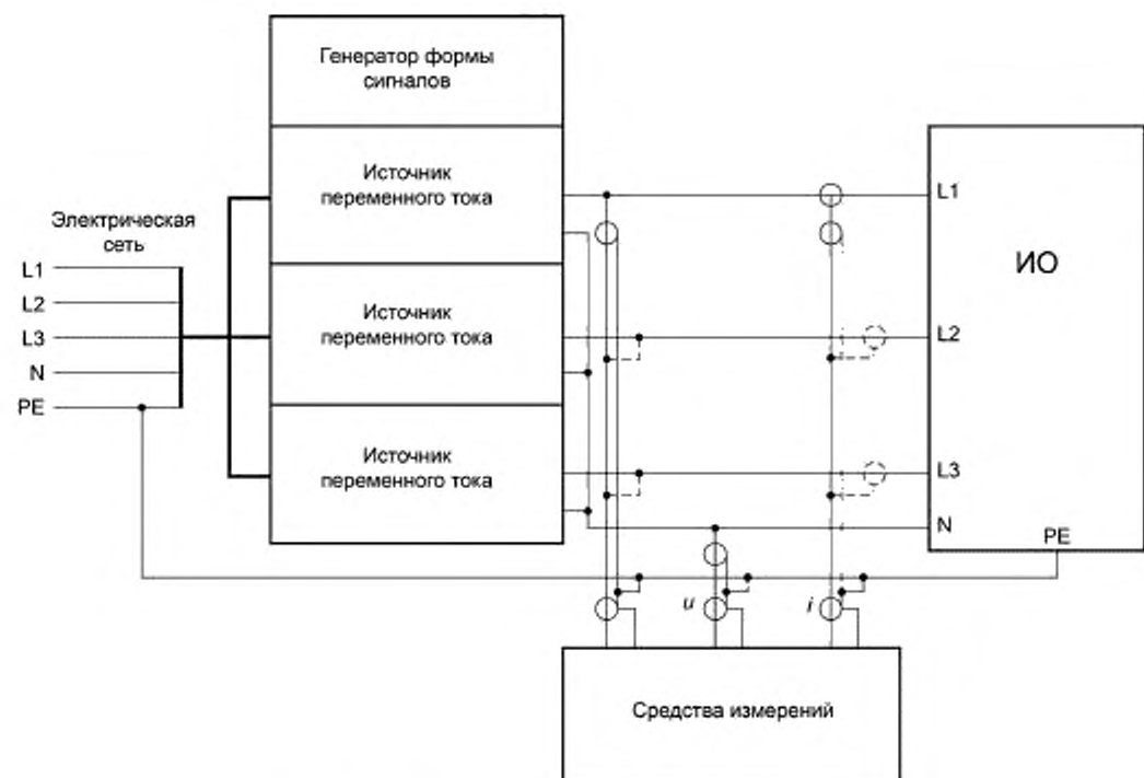
Рисунок 3 — Пример испытательной установки для трехфазной сети
