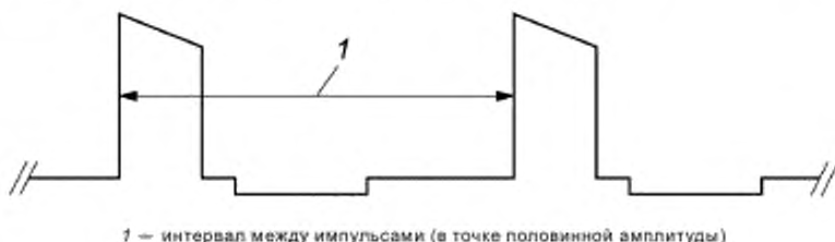
Рисунок 104 — Измерение интервала импульса для расчета частоты
