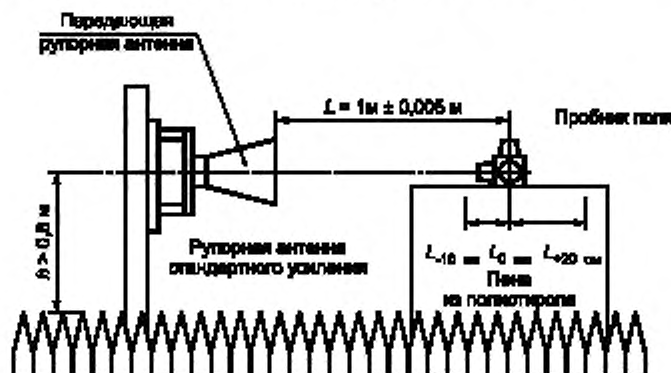
Рисунок 1.3 — Испытательная установка для валидации камеры
