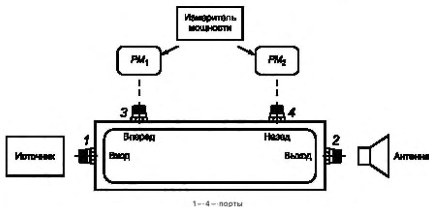
Рисунок 1.2 — Установка для измерения мощности, поступающей к передающему устройству
