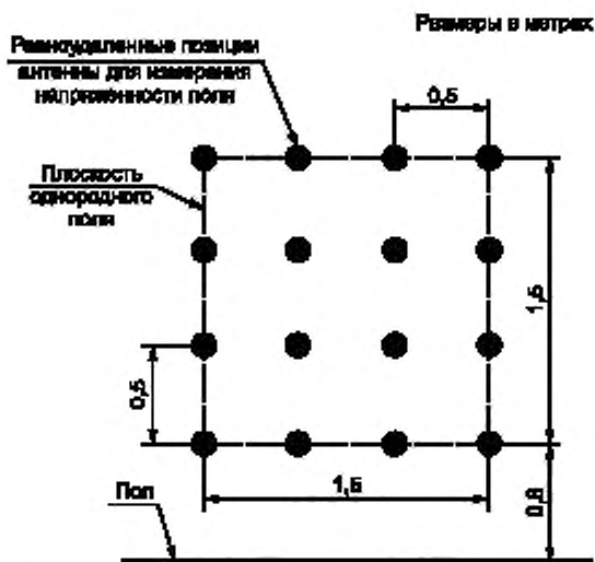
Рисунок 4 — Калибровка поля; размеры плоскости однородного поля
