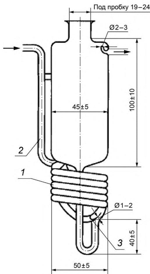
Рисунок 5 — Абсорбер
