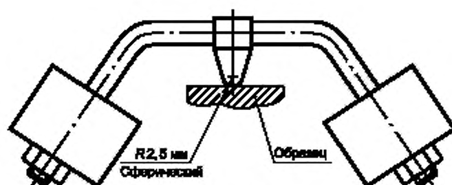
Рисунок 6 — Приспособление для вдавливания шарика
