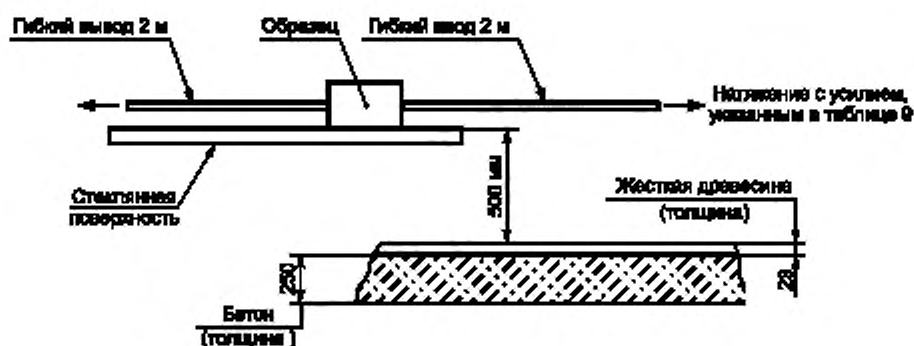
Рисунок 4 — Испытание на удар отдельно стоящих управляющих устройств
