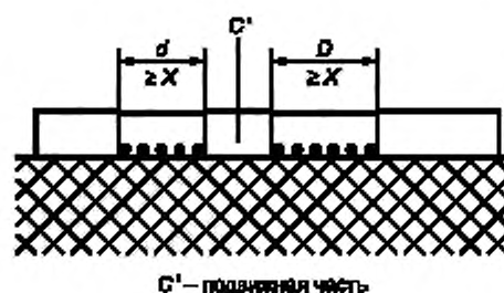
Рисунок В.9 — Узкое углубление
