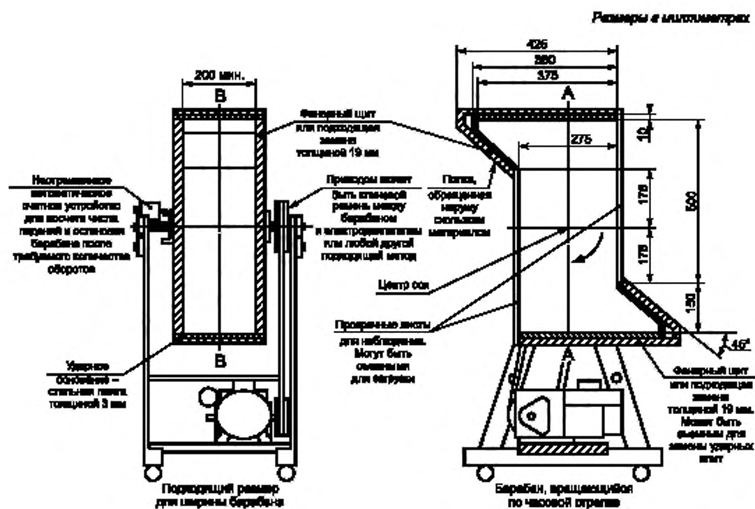
Рисунок 5 — Вращающийся барабан
