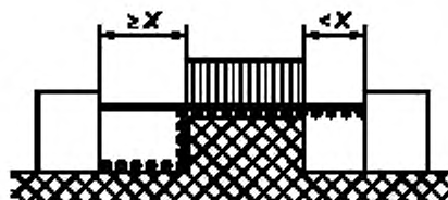
Рисунок В.6 — Несклеенное соединение с широкой прорезью
