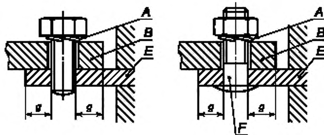
b) Зажимы под наконечник
