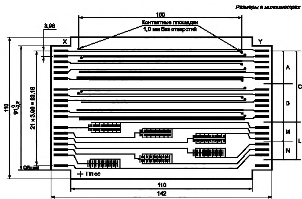
Рисунок Q.1 — Испытательный образец
