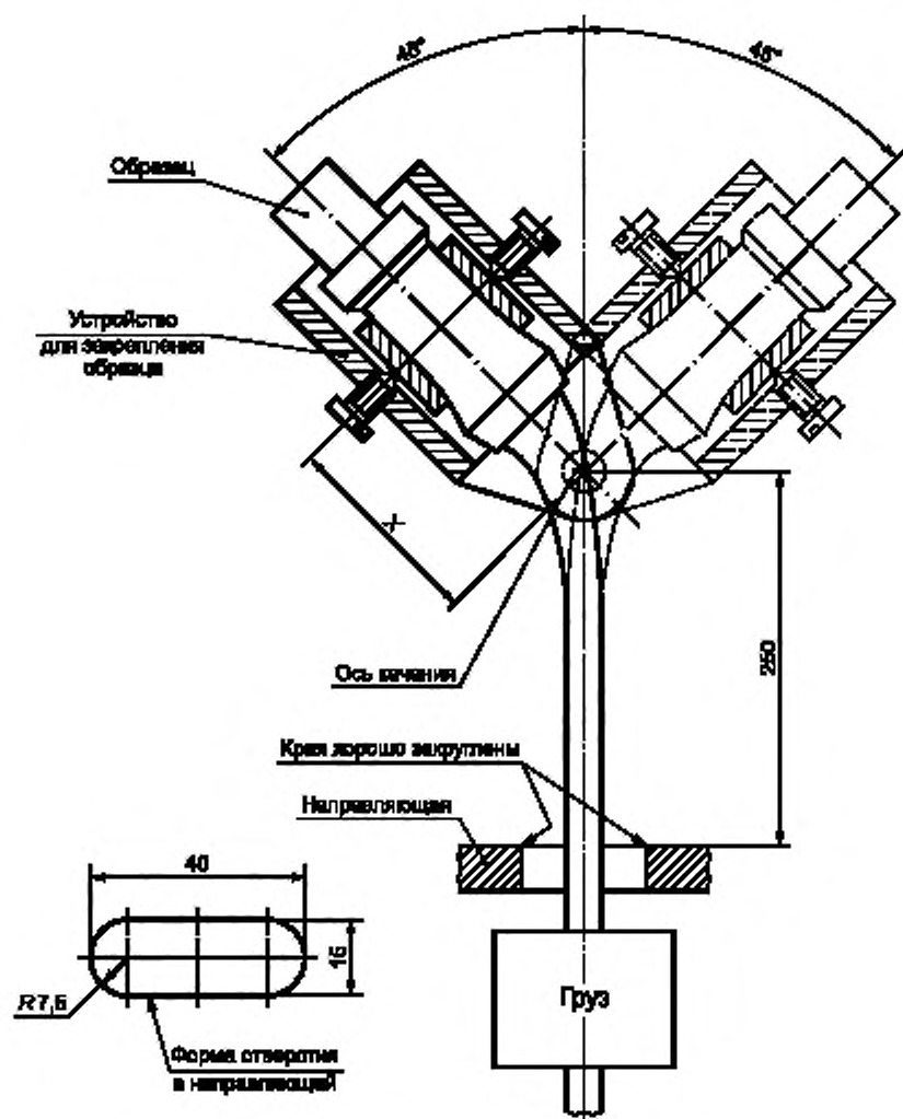
Рисунок 9 — Приспособление для испытания на изгиб
