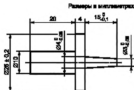
Рисунок 1 — Испытательный штырь
