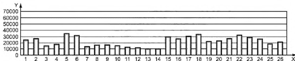
Рисунок А.1 — Результат содержания грибов (КОЕ/г DG-18) в полистироле по время испытаний (номера от 1 до 26 обозначают лаборатории и параллельные пробы)
