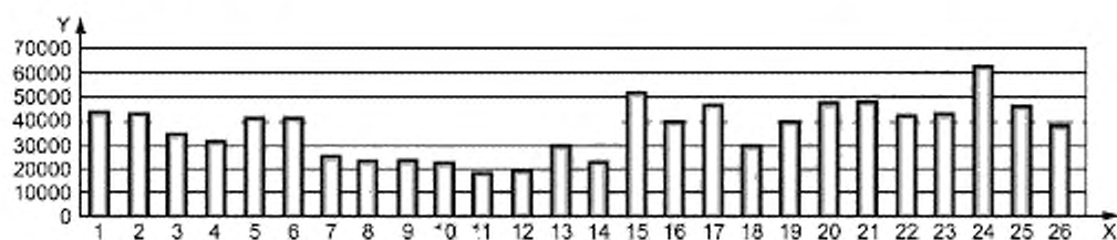
Рисунок А.2 — Результат содержания грибов (КОЕ/г MEA) в полистироле во время испытаний (номера от 1 до 26 обозначают лаборатории и параллельные пробы)
