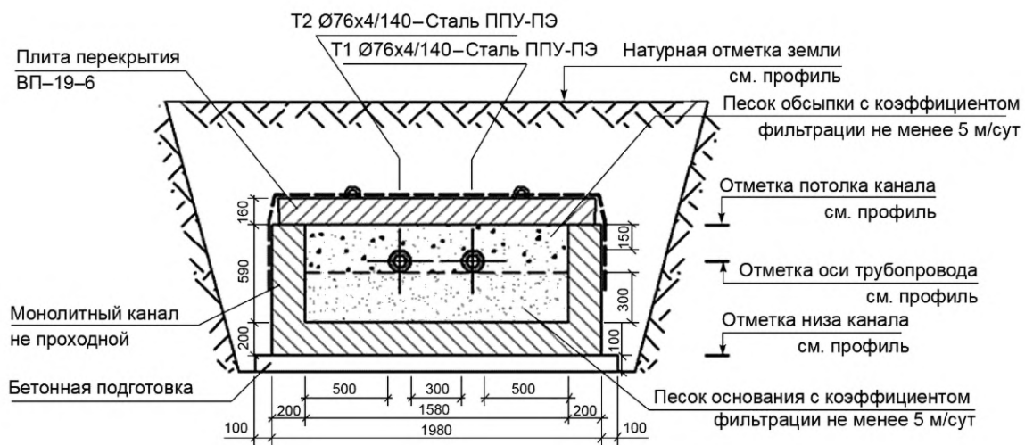
Рисунок Г.4 — Поперечный разрез при прокладке сетей в засыпном канале
