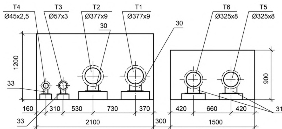
Рисунок Г.1 — Поперечный разрез при подземной прокладке
