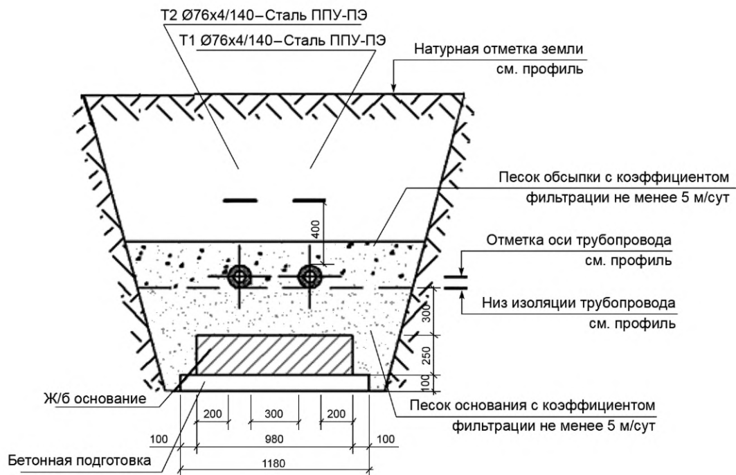
Рисунок Г.5 — Поперечный разрез. Бесканальная прокладка в траншее по бетонной подготовке
