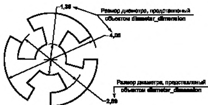
Рисунок 4 – Размер диаметра
