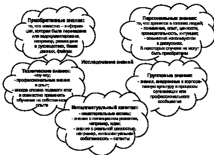
Рисунок 1 — Типы знаний
