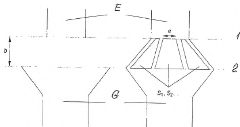
1 – слив; 2 – уровень перелива; E – сливное отверстие; G – дренажное отверстие; S1, S2 ... – Входные отверстия для воздуха с поперечным сечением для прохода воздуха; e – наименьший размер для расчета поперечного сечения; b – высота воздушного зазора
