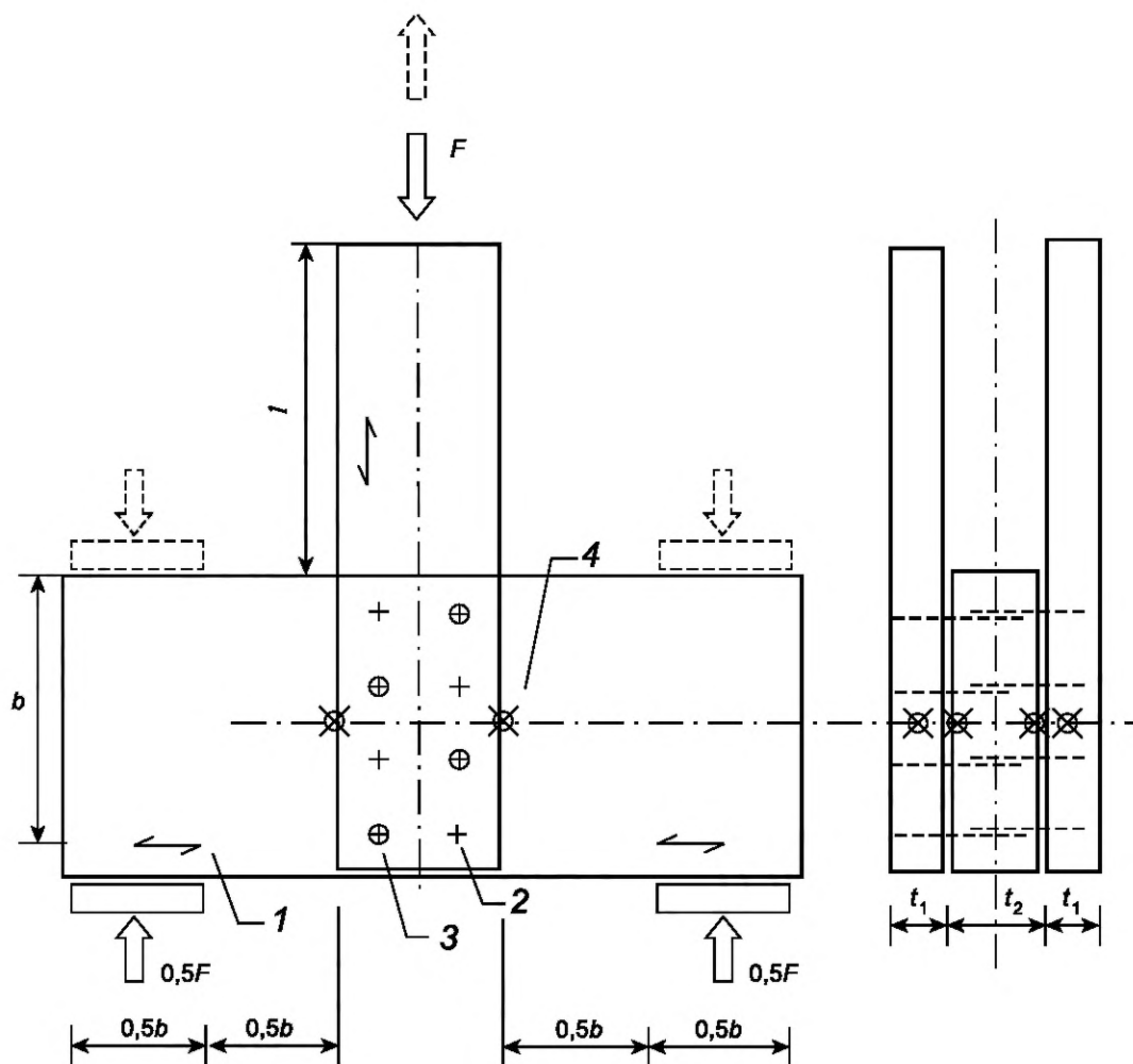
1 — направление волокон; 2 — невыступающая часть крепежа; 3 — выступающая часть крепежа; 4 — \oplus точки измерения смещений; l — смещение элементов; t_1 — ширина крайнего элемента; t_2 — ширина среднего элемента
