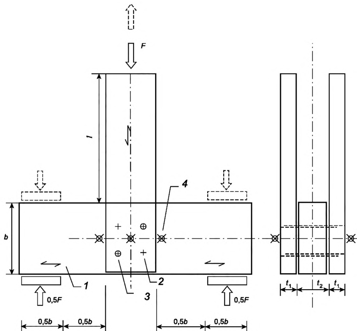
1 — направление волокон; 2 — невыступающая часть крепежа; 3 — выступающая часть крепежа; 4 — \oplus точки измерения перемещений; l — величина смещения элементов; t_1 — ширина крайнего элемента; t_2 — ширина среднего элемента
