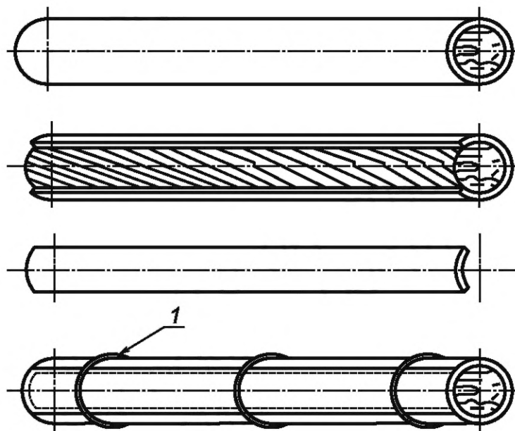
Рисунок В.1 — Специально подготовленные испытываемые образцы
