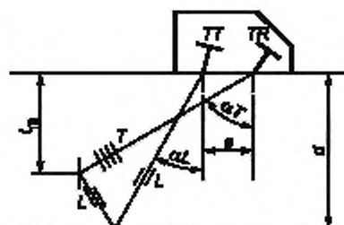
TT — излучающий активный элемент; TR — принимающий активный элемент; e — расстояние между точками выхода активных элементов; d — толщина материала; t_m — контролируемая глубина точки пересечения; L — путь продольной волны; T — путь поперечной волны
