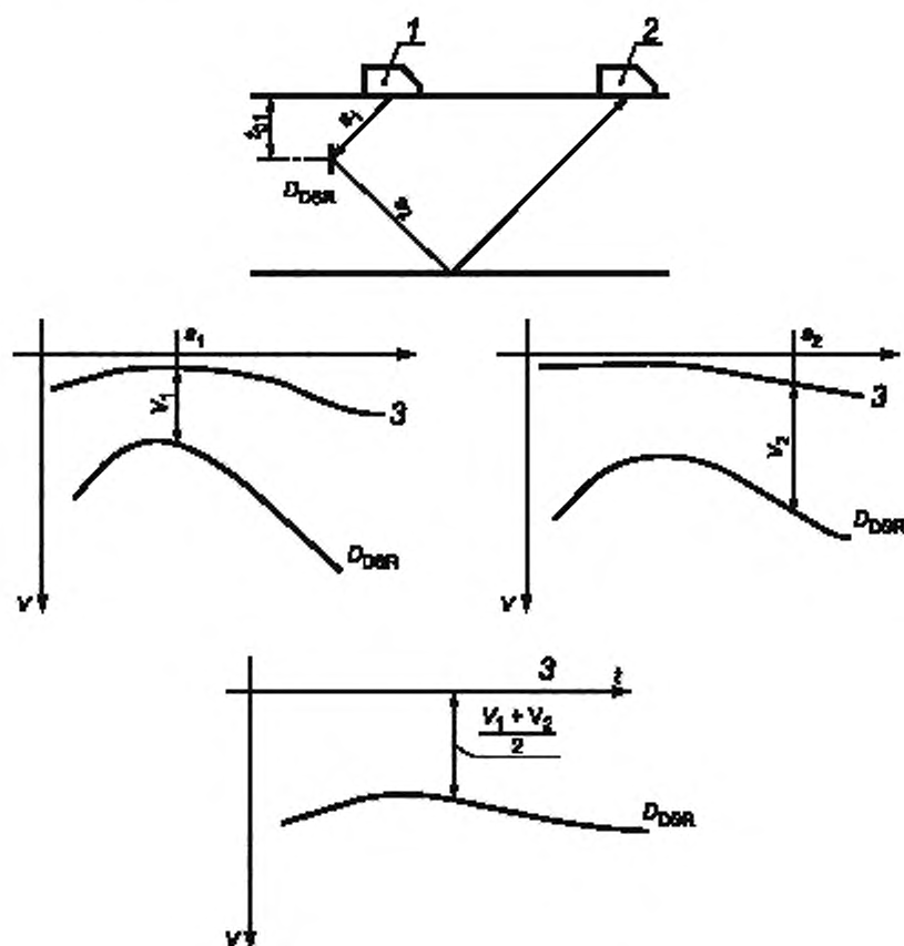
D_{DSR} — диаметр плоского отражателя; s — длина пути звука; l — глубина дефекта от сканируемой поверхности; V — изменение усиления; 1, 2 — преобразователи №№ 1, 2; 3 — донная поверхность
