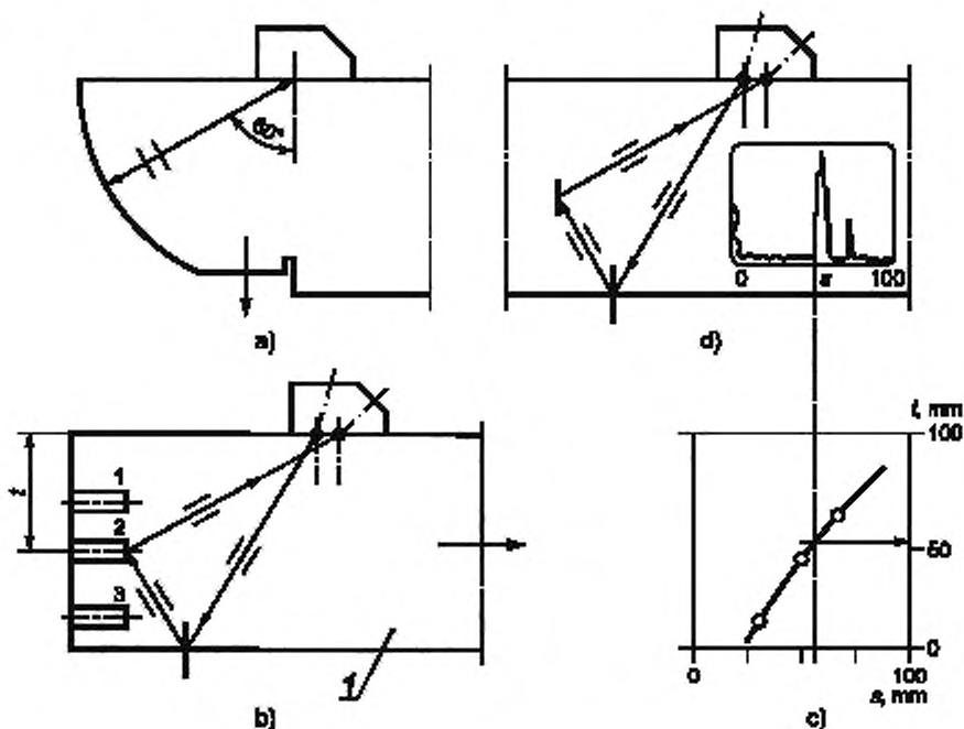
1 — настроечный образец; t — глубина дефекта от сканируемой поверхности; L — длина пути звука
