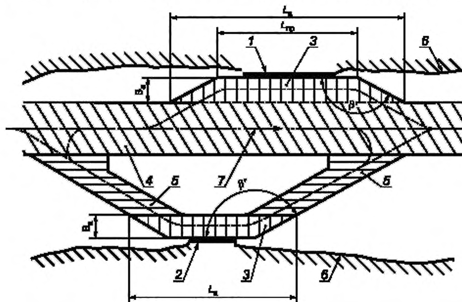
1 — причалы, расположенные в непосредственной близости от судового хода; 2 — причал, расположенный в стороне от судового хода; 3 — акватория причалов; 4 — транзитный или местный судоводительский ход; 5 — водные подходы к акватории причалов; 6 — береговая полоса; 7 — направление течения
