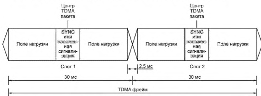
Рисунок А.4 — TDMA фрейм от источника MC
