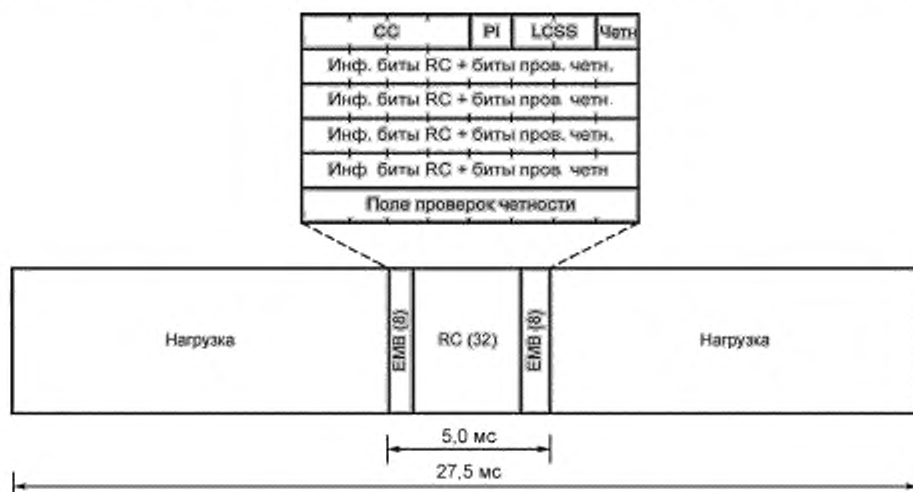
Рисунок А.19 — Формат пакета реверсного канала
