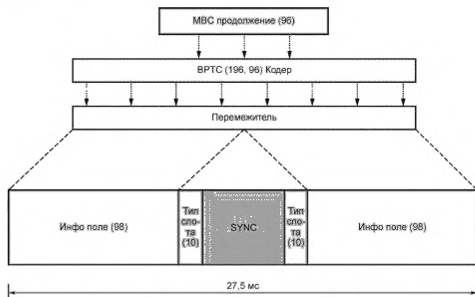
Рисунок A.27 — Формат пакета промежуточного MBC сообщения
