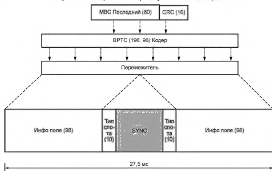
Рисунок A.28 — Формат последнего блока MBC сообщения
