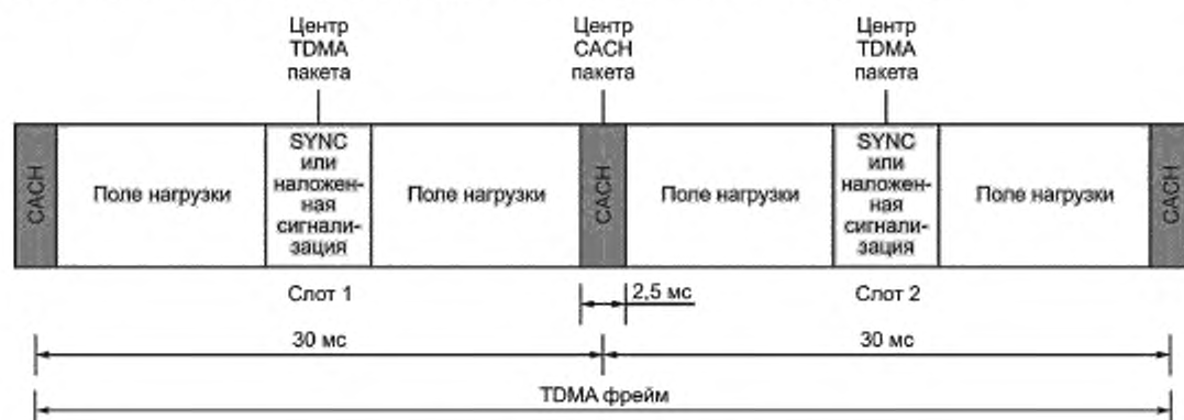
Рисунок А.5 — Структура TDMA фрейма от источника BC
