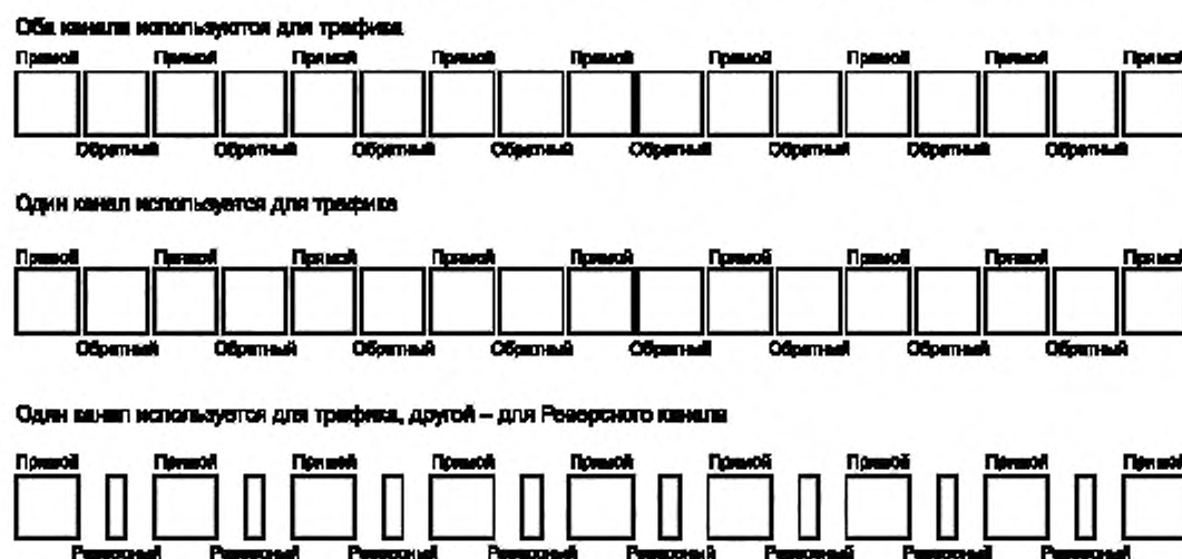
Рисунок А.10 — Двухнаправленный канал
