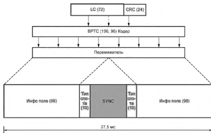
Рисунок A.23 — Формат пакета «Окончание LC»
