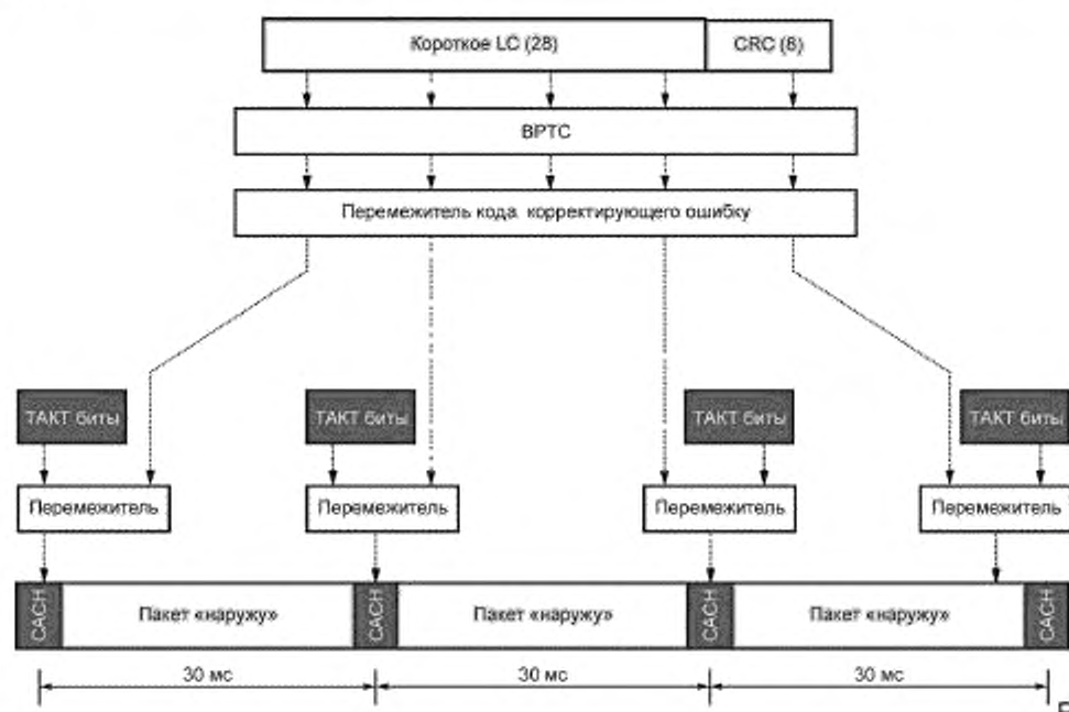
Рисунок A.24 — Короткое LC сообщение в составе CACH
