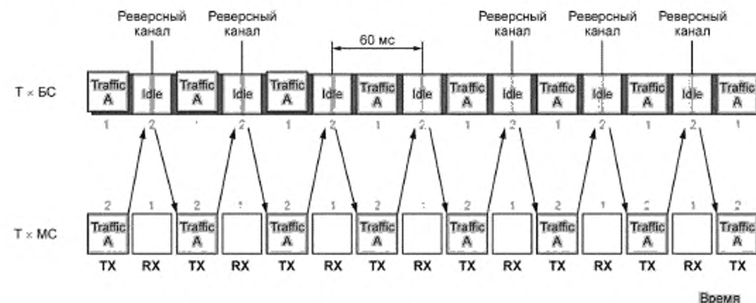
Рисунок A.15 — Синхронизация назначенного реверсного канала
