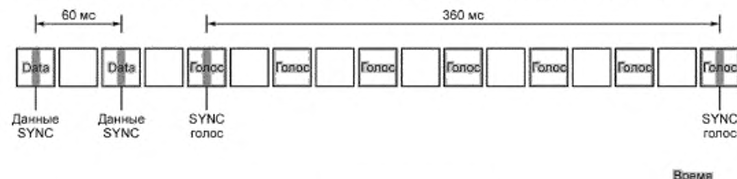
Рисунок A.6 — Синхронизация канала от МС к БС
