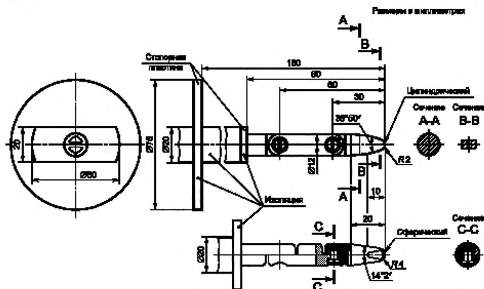
Рисунок 2 — Шарнирный щуп
