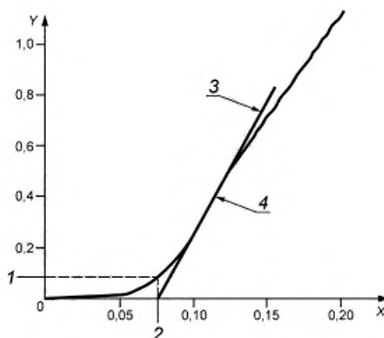
X = t, c; Y = V, c; 1 = V_E = 0,084 \text{ л}; 2 = t_0 = 0,075 \text{ с}; 3 — касательная, проведенная через точку ПОС с тангенсом наклона, равным ПОС; 4 — ПОС = 10,8 л/с при 0,114 с
