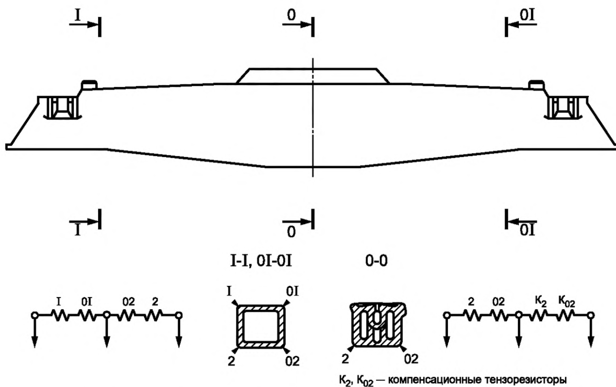
Рисунок Б.2 — Схема установки и соединения тензорезисторов для определения коэффициента динамической добавки обрессоренных частей в сечениях наддрессорной балки тележки грузового вагона
