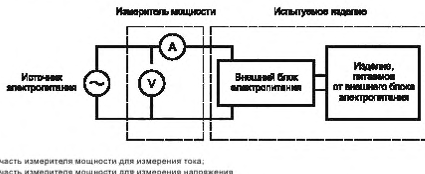
Рисунок В.2 — Схема расположения прибора, питаемого от внешнего источника питания для маломощных нагрузок
