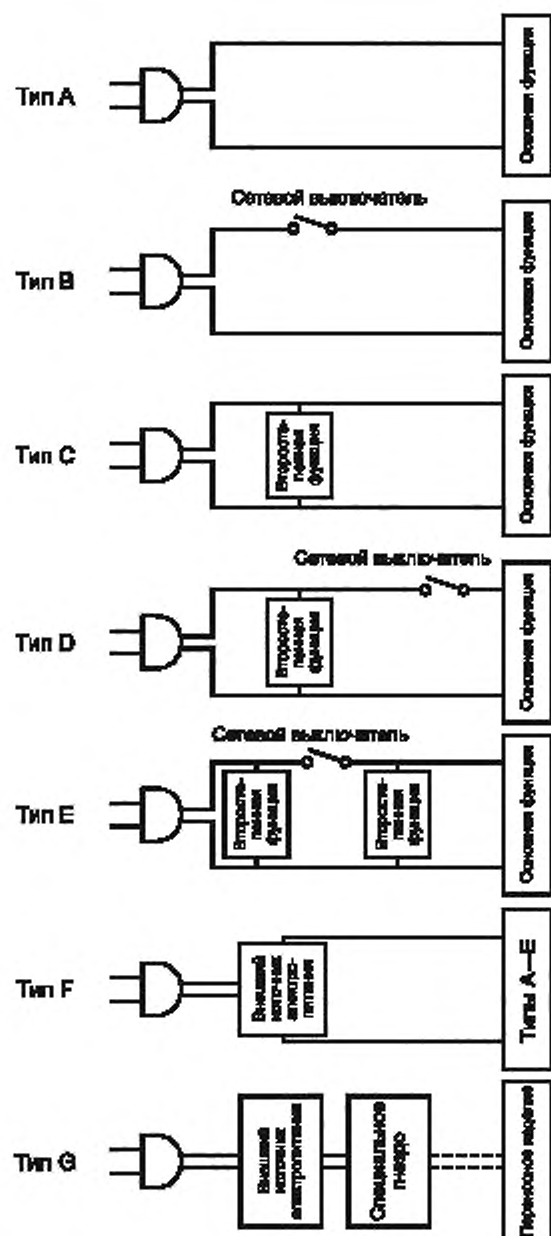
Рисунок A.1 — Принципиальные схемы типов приборов
