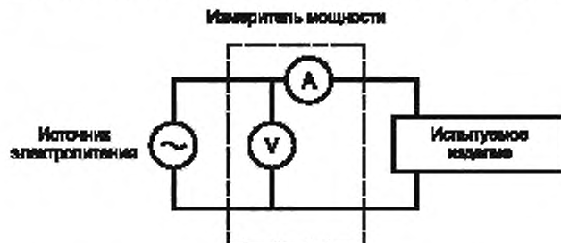
Рисунок В.1 — Схема расположения для приборов, питаемых непосредственно от источника питания переменного тока для маломощных нагрузок
