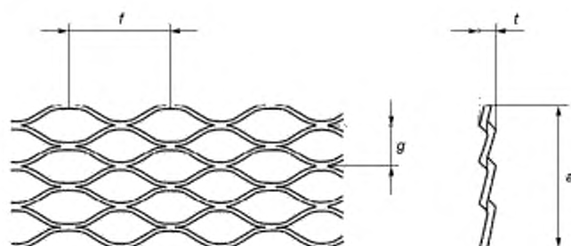
Рисунок 5.4 — Просечно-вытяжная сетка
