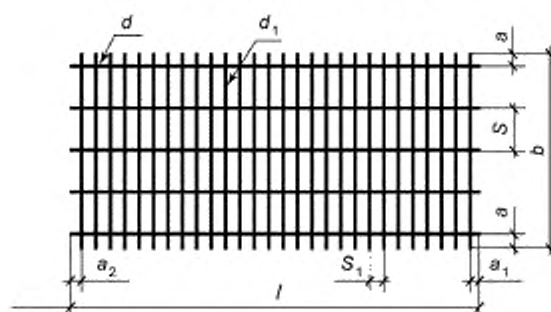
Рисунок 5.6 — Сетка с прямоугольной ячейкой
