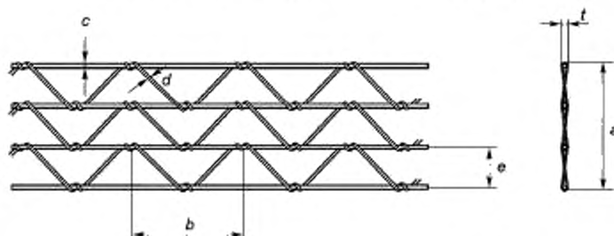
Рисунок 5.3 — Сетка с плетеной конфигурацией
