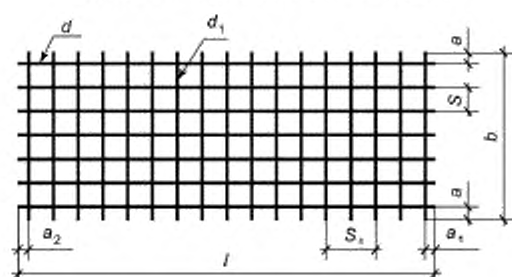
Рисунок 5.5 — Сетка с квадратной ячейкой
