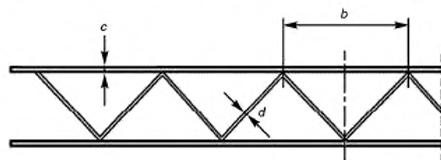
Рисунок 5.2 — Сетка с фахверковой конфигурацией
