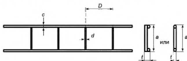
Рисунок 5.1 — Сетка с решетчатой конфигурацией
