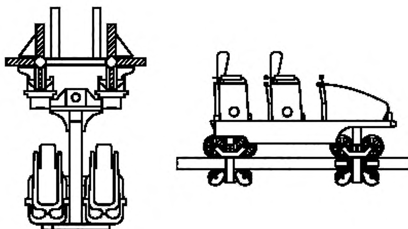
а) Атракцион с направляющими
