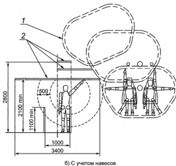
1 — контур безопасности пассажирского модуля; 2 — навес
