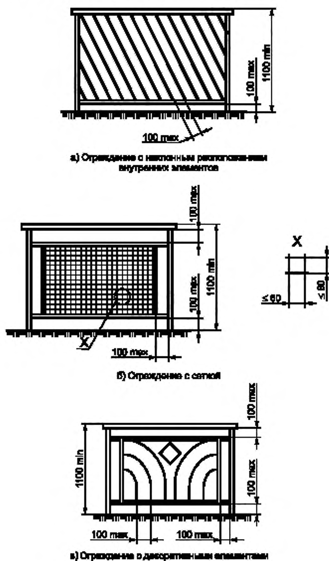
Рисунок 4 — Типы ограждений
