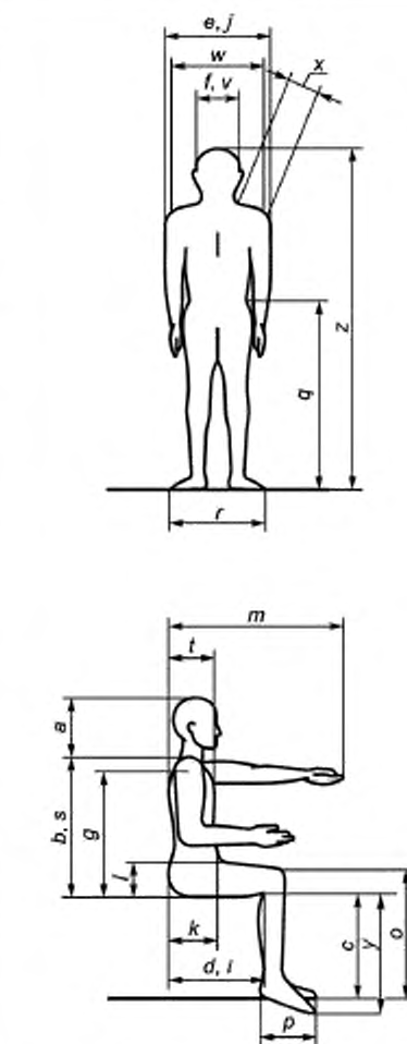
Рисунок Д.1 — Размеры тела (таблица Д.2)
