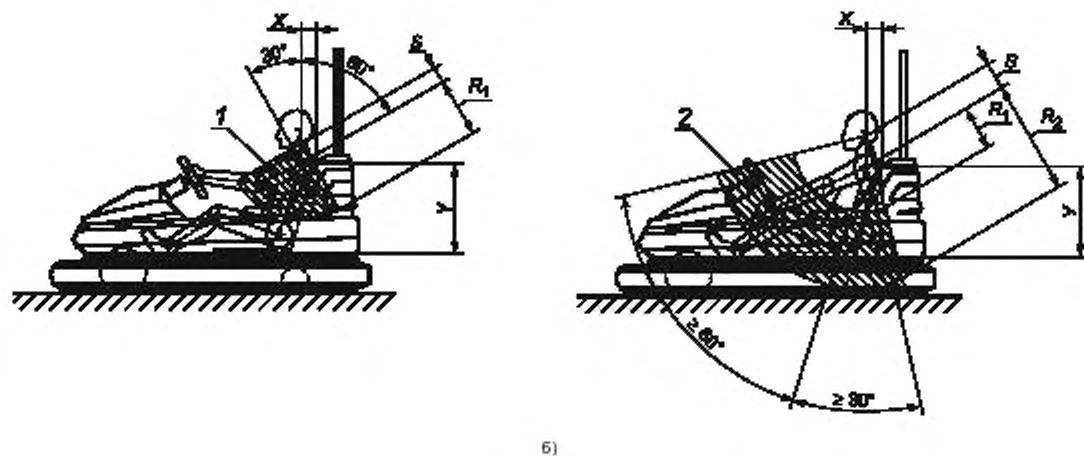
Рисунок 15 — Сталкивающиеся электромобили
