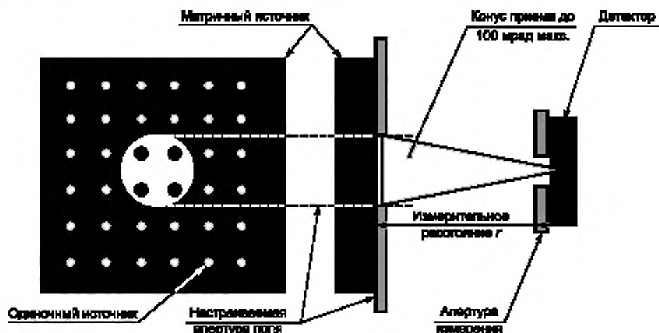
10а -- Геометрия измерения для доступного источника
