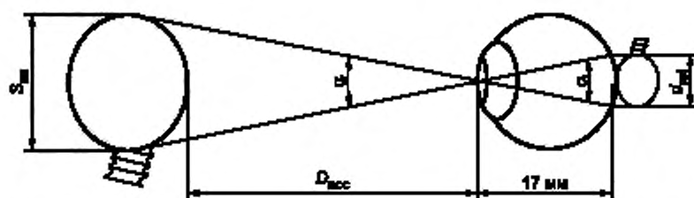
6а — Стягиваемый угол ( \alpha ) и размер видимого источника ( s_{вс} ) некогерентного или диффузного источника
