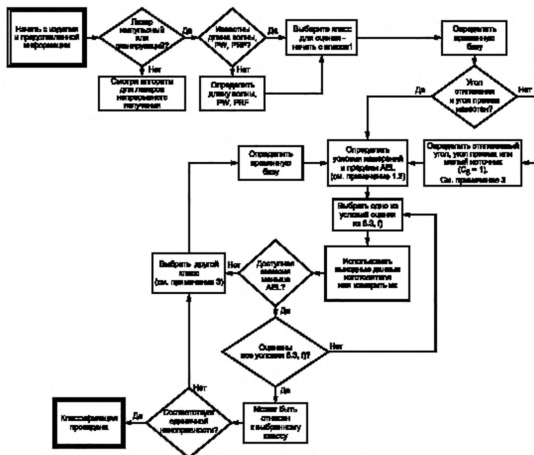
Рисунок 2 — Алгоритм классификации импульсных лазеров
