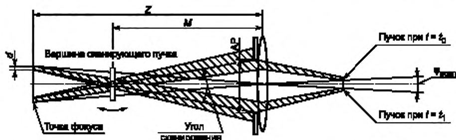
Рисунок 13 — Изображение сканирующего видимого источника, находящегося за вершиной сканирующего пучка
