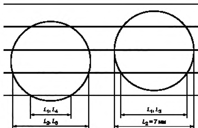
Рисунок А.1 — Несколько линий раstra, пересекающих измерительную апертуру на расстоянии от вершины сканирования, при котором коэффициент C_6 = 1
