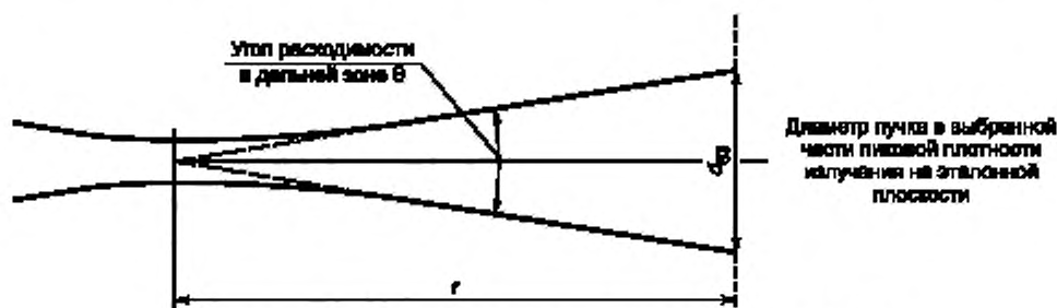
Рисунок 7 — Местоположение перетяжки пучка при Гауссовом пучке
