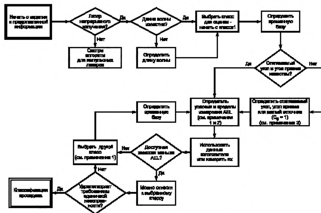
Рисунок 1 — Алгоритм классификации лазеров непрерывного излучения
