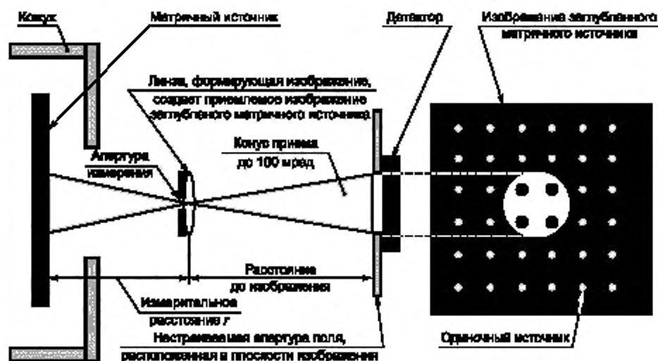
10b -- Геометрия измерения для углубленного источника
