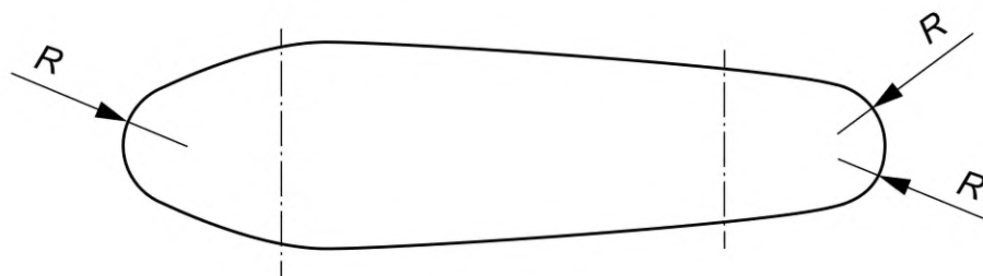
Рисунок 2 — Дека скейтборда
