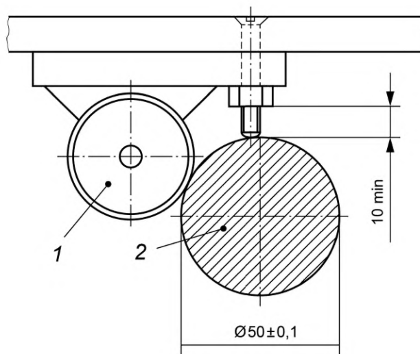
1 — ролик; 2 — испытательный цилиндр
