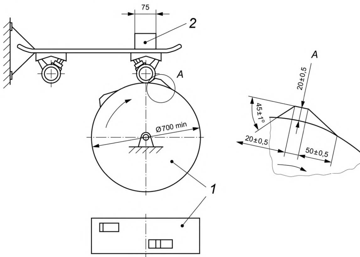
1 — испытательный цилиндр с выступами; 2 — груз
