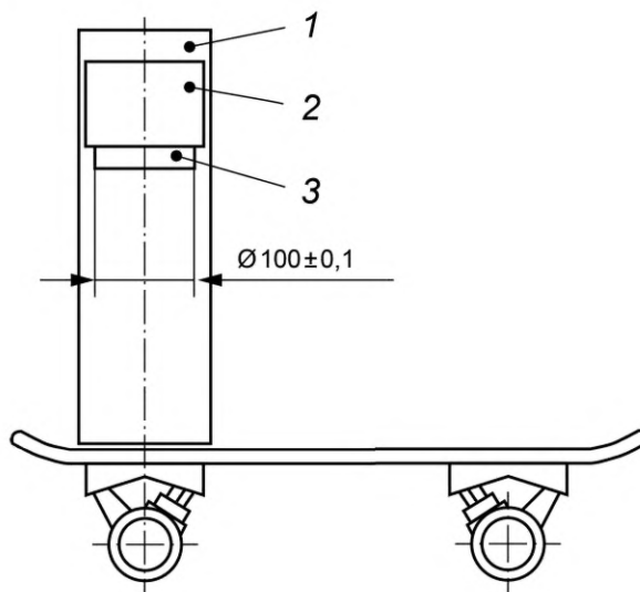
1 — направляющая труба; 2 — груз; 3 — резиновая накладка
