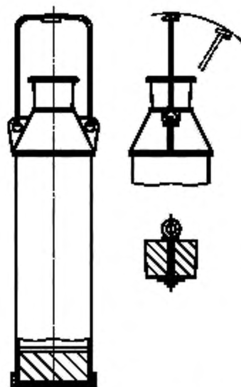
Рисунок А.7 — Простой утяжеленный металлический сосуд
