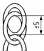
Рисунок 9 — Максимальные отверстия в цепях для качелей
