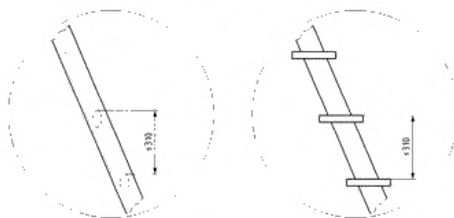
б) детали лестницы со ступенями
