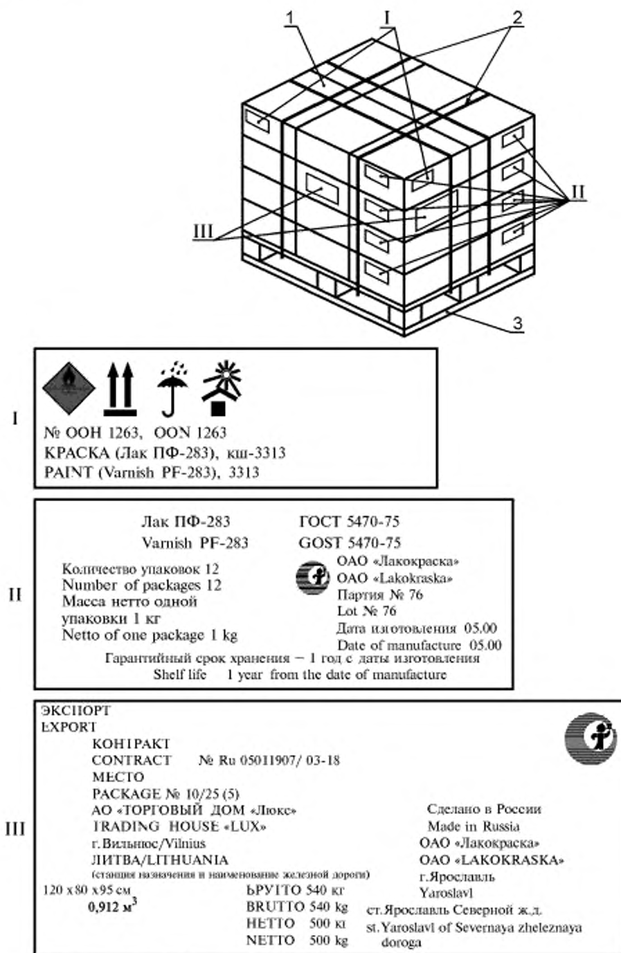
Рисунок К.2 — Маркировка продукции в картонных ящиках, сформированных в транспортный пакет
