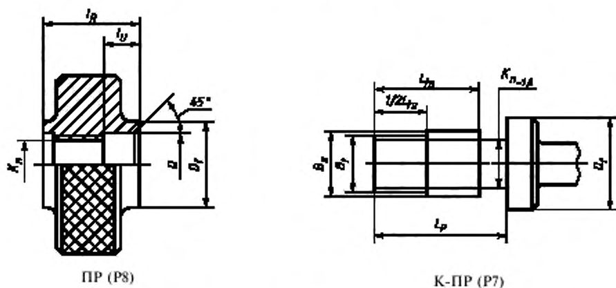
Рисунок Д.1 — Основные размеры калибров PR (P8) и К-PR (P7) для контроля резьбы ниппеля
