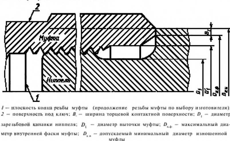
Рисунок 11 — Сопрягаемые элементы ниппелей штанг и муфт к ним
