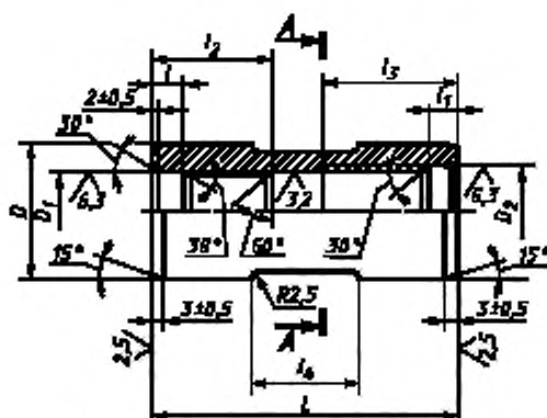
Рисунок 5 — Переводные муфты
