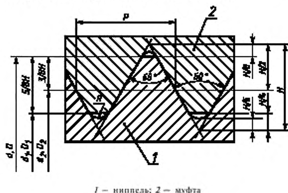
Рисунок 9 — Номинальный профиль резьбы
