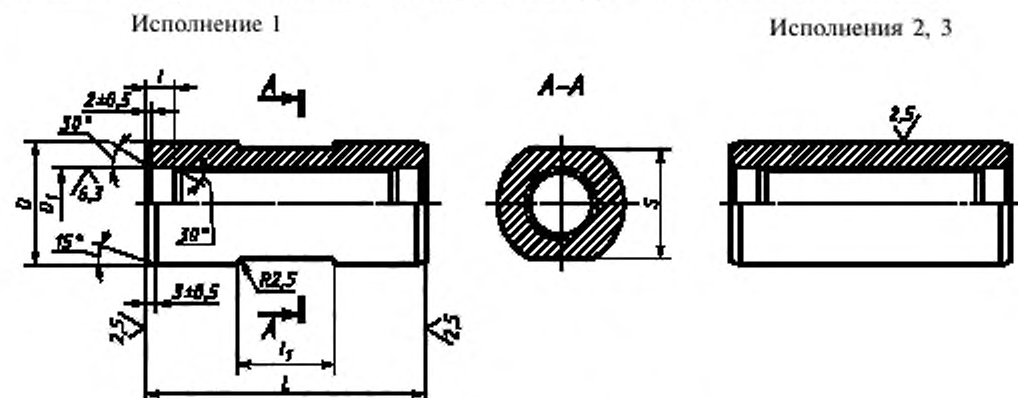
Рисунок 4 — Соединительные муфты
