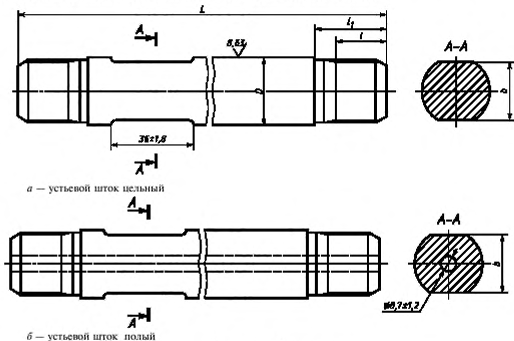
Рисунок 6 — Устьевой шток
