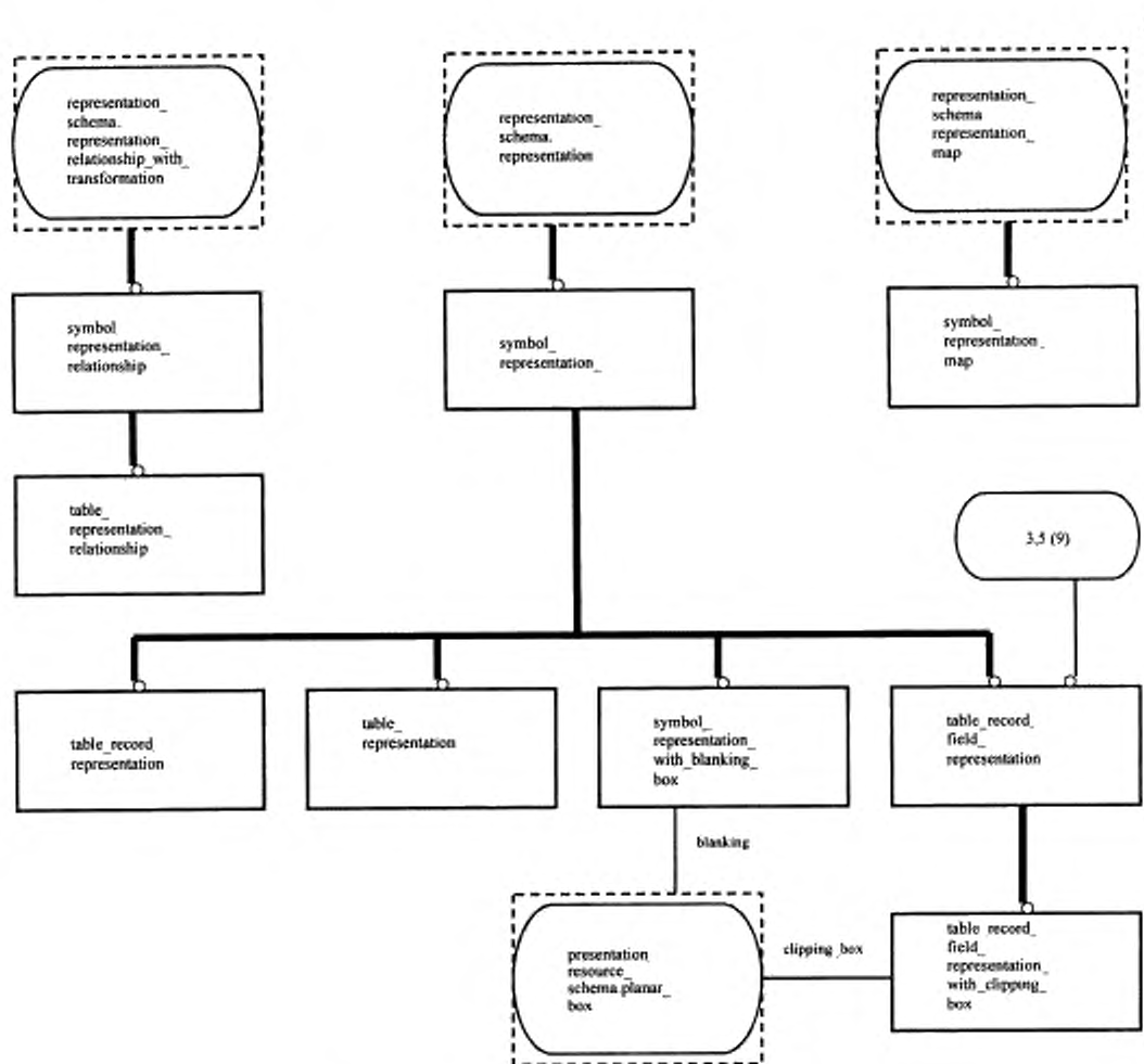
Рисунок Е.10 — EXPRESS-G диаграмма presentation_definition_schema 3 из 9
