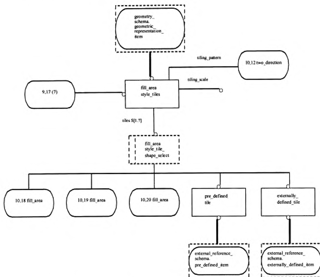
Рисунок Е.25 — EXPRESS-G диаграмма presentation_appearance_schema 9 из 21
