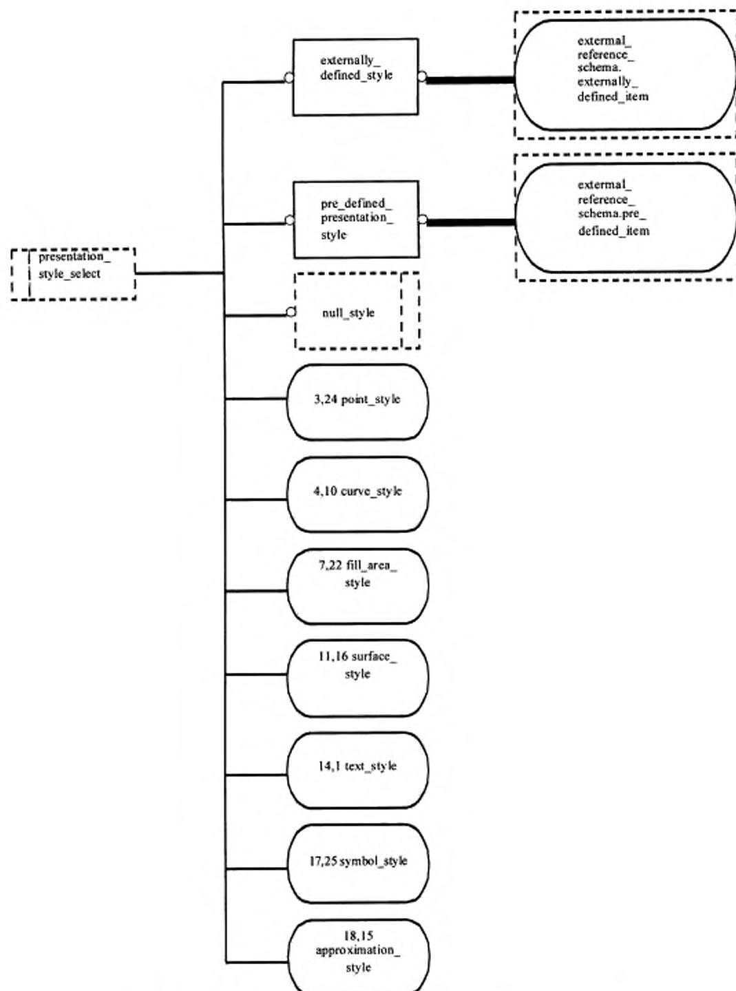
Рисунок Е.18 — EXPRESS-G диаграмма presentation_appearance_schema 2 из 21
