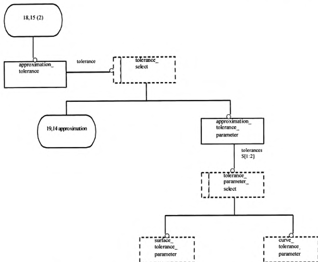
Рисунок Е.34 — EXPRESS-G диаграмма presentation_appearance_schema 18 из 21
