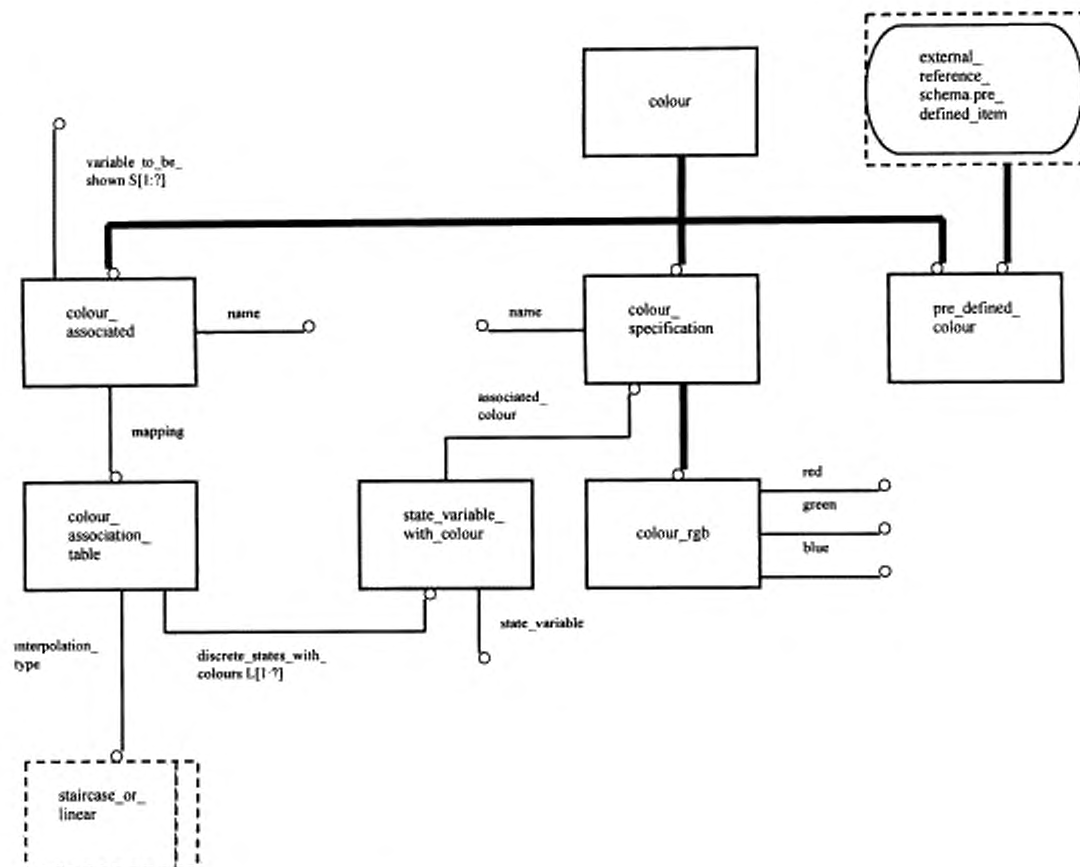
Рисунок Е.41 — EXPRESS-G диаграмма presentation_resource_schema 4 из 5
