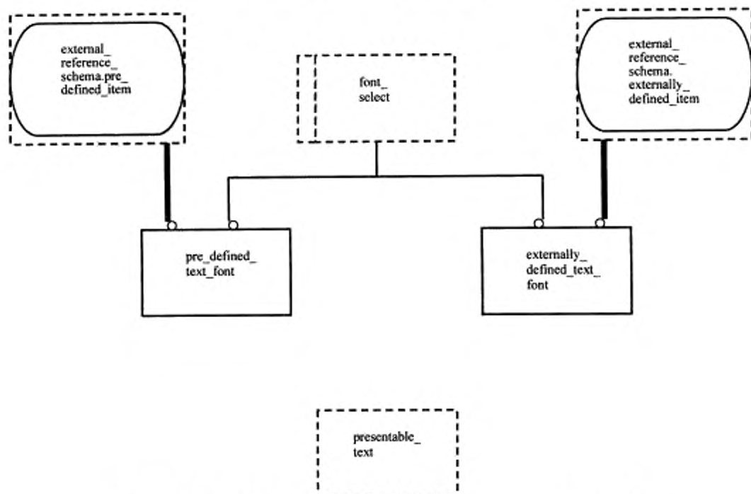
Рисунок Е.40 — EXPRESS-G диаграмма presentation_resource_schema 3 из 5
