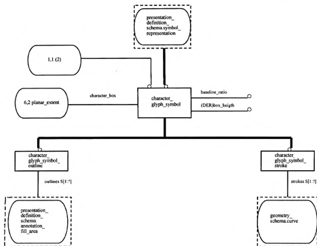
Рисунок E.38 — EXPRESS-G диаграмма presentation_resource_schema 1 из 5
