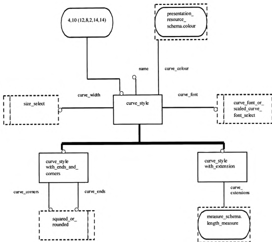
Рисунок Е.20 — EXPRESS-G диаграмма presentation_appearance_schema 4 из 21
