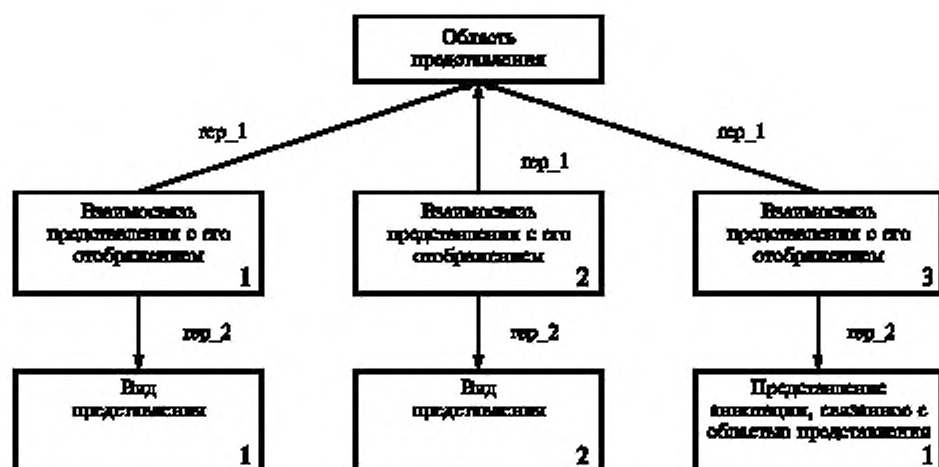
Рисунок 3 — Отображение иерархии представления на экземпляры объектов
