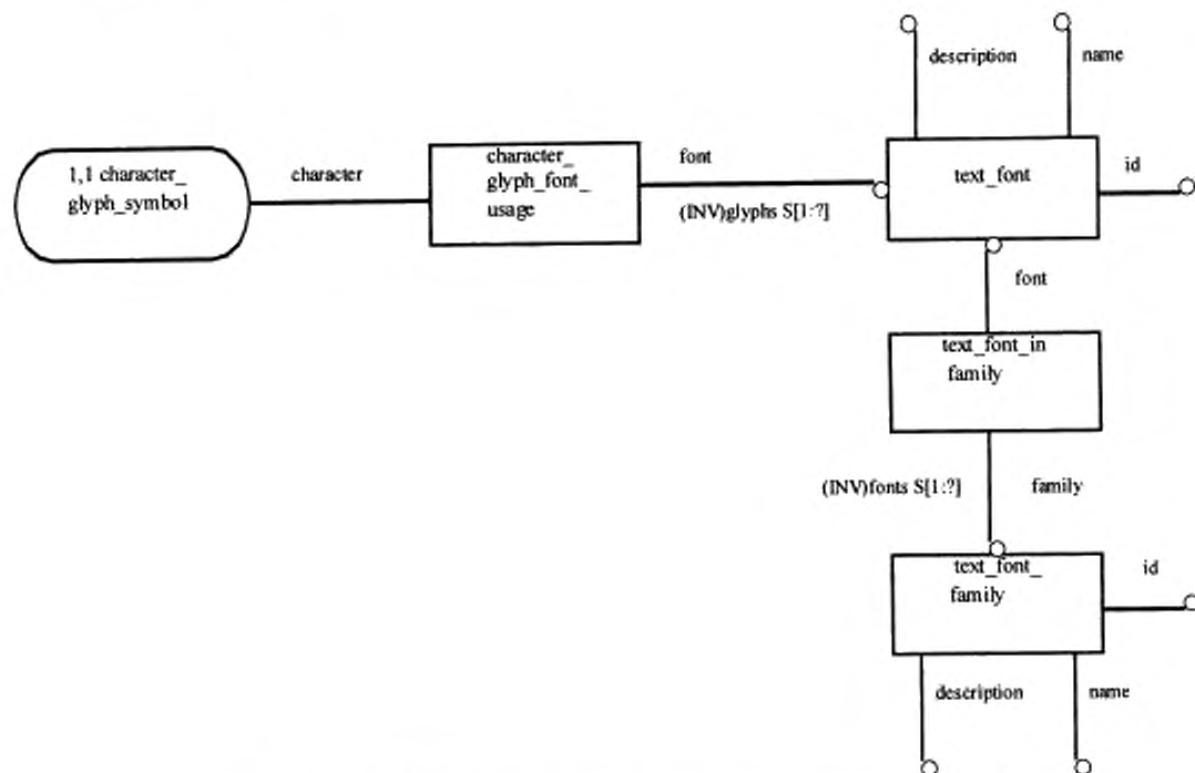
Рисунок Е.39 — EXPRESS-G диаграмма presentation_resource_schema 2 из 5
