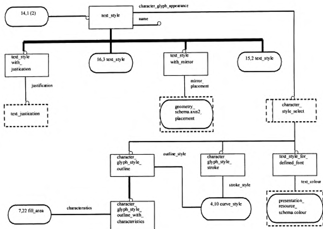
Рисунок E.30 — EXPRESS-G диаграмма presentation_appearance_schema 14 из 21
