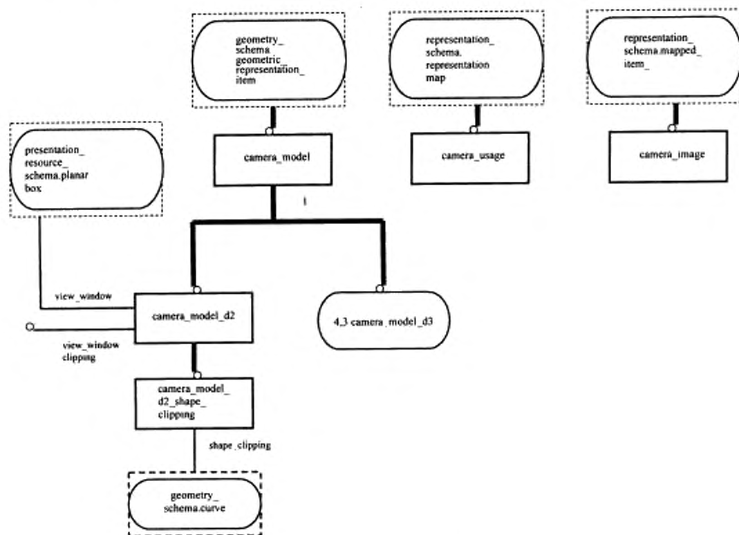
Рисунок Е.3 — EXPRESS-G диаграмма presentation_organization_schema 3 из 7
