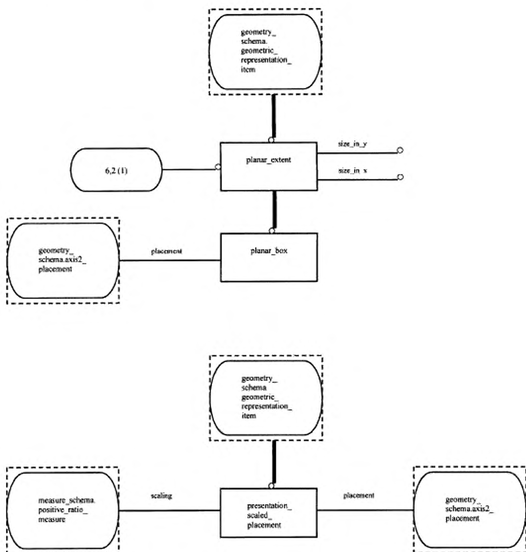
Рисунок Е.42 — EXPRESS-G диаграмма presentation_resource_schema 5 из 5
