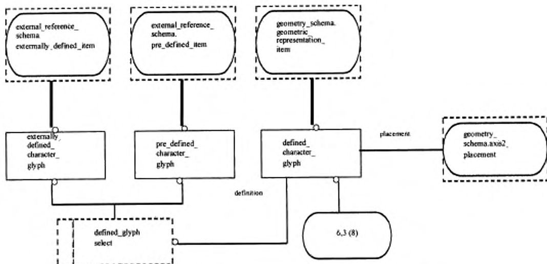
Рисунок Е.13 — EXPRESS-G диаграмма presentation_definition_schema 6 из 9
