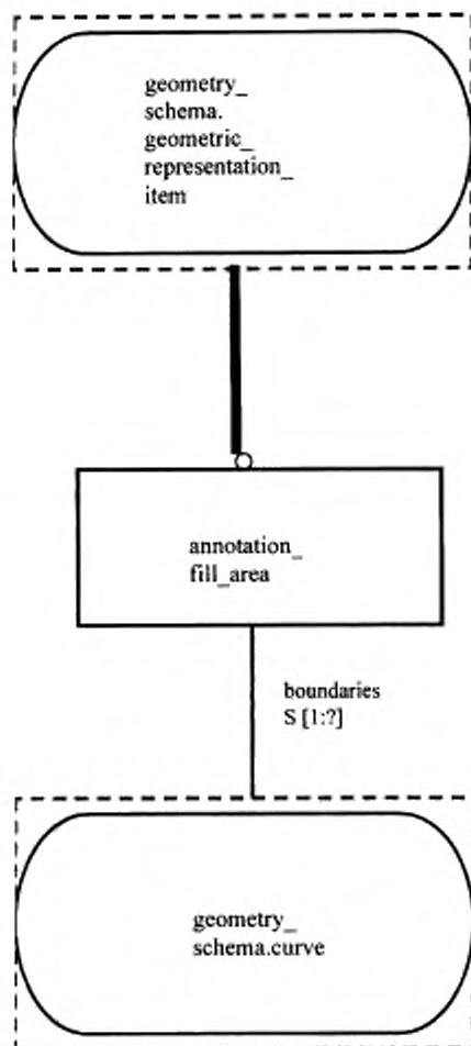
Рисунок Е.8 — EXPRESS-G диаграмма presentation_definition_schema 1 из 9
