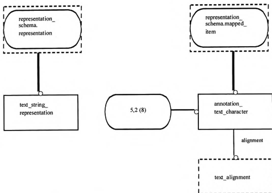
Рисунок Е.12 — EXPRESS-G диаграмма presentation_definition_schema 5 из 9
