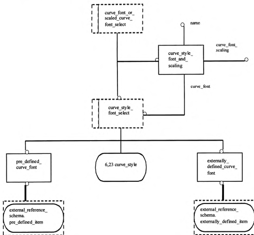
Рисунок Е.21 — EXPRESS-G диаграмма presentation_appearance_schema 5 из 21
