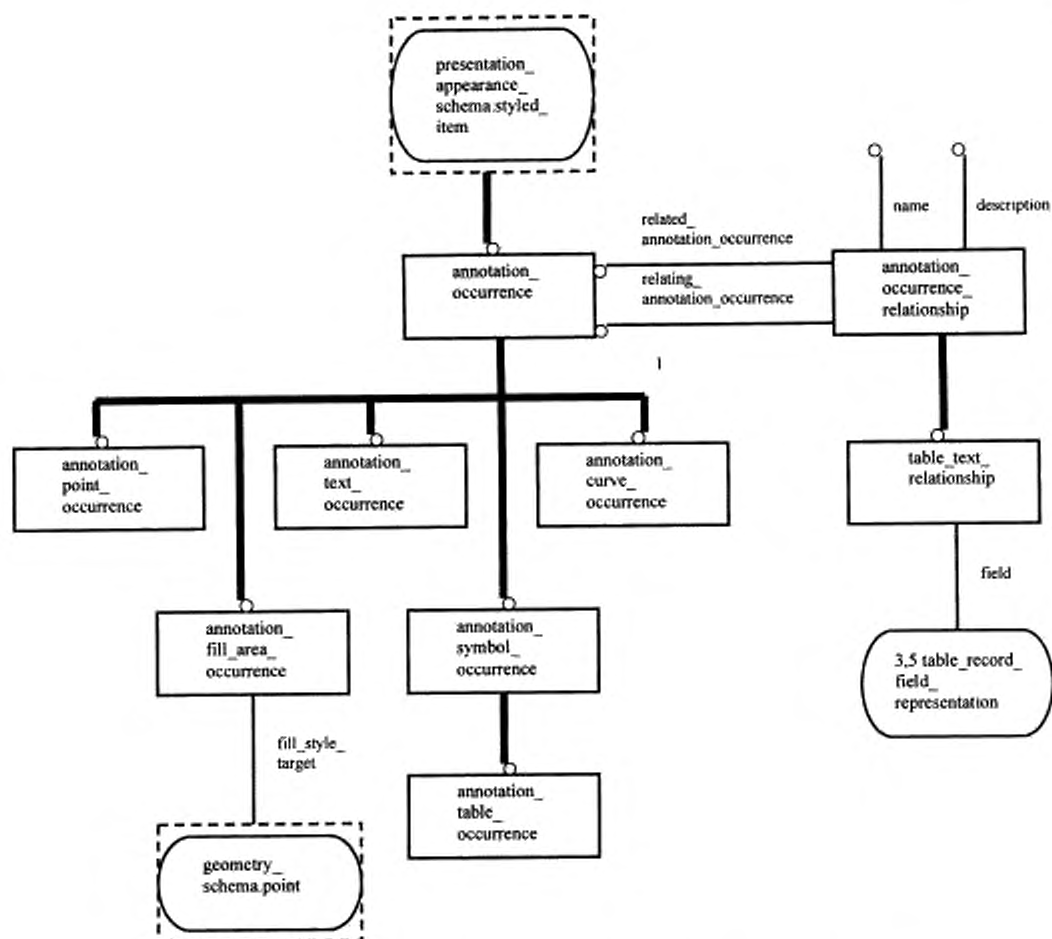
Рисунок Е.16 — EXPRESS-G диаграмма presentation_definition_schema 9 из 9
