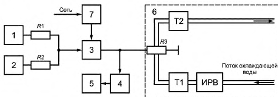
1, 2 — генераторы сигналов НЧ; 3 — передатчик; 4 — элемент связи; 5 — анализатор спектра ВЧ; 6 — эквивалент антенны; R3 — водохлаждаемый согласованный резистор; T1, T2 — термометры воды на входе и выходе системы охлаждения; ИПВ — измеритель расхода воды; 7 — ваттметр (измерительный комплект для измерения потребляемой мощности); R1, R2 — резисторы сопротивлением (6,8 \pm 0,34) \text{ кОм}
