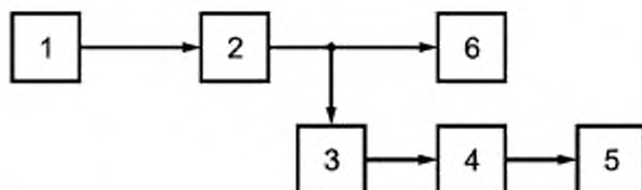
Рисунок 22 — Схема измерения контрольной ширины полосы радиочастот и спектра внеполосных радиокосебаний в телеграфных режимах работы
