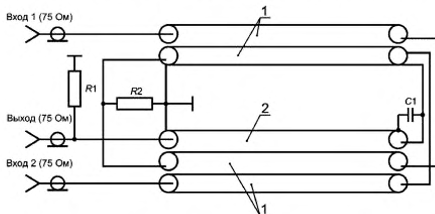
1 — коаксиальный кабель типа РК-75-1,5-22; 2 — коаксиальный кабель типа КВФ-37; R1 — резистор сопротивлением 75 Ом; R2 — резистор сопротивлением 37,5 Ом; C1 — конденсатор 16 пФ
