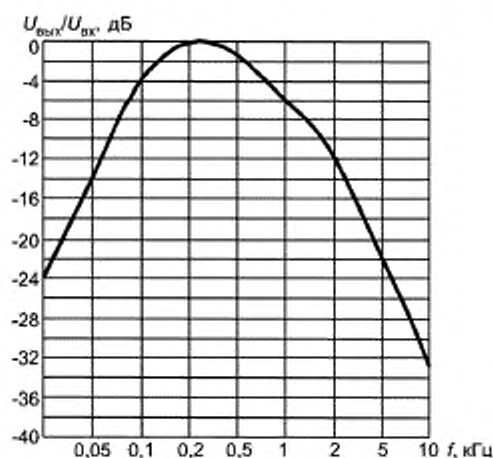
Рисунок Е.1 — АЧХ фильтра, формирующего спектр вещательного сигнала
