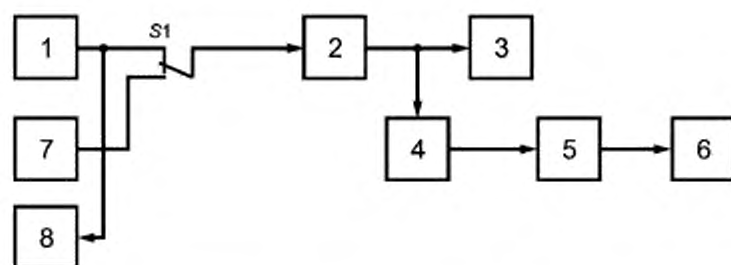
1 — генератор сигналов НЧ; 2 — передатчик; 3 — эквивалент антенны; 4 — элемент связи; 5 — УОП передатчика; 6 — милливольметр НЧ; 7 — экранированный резистор сопротивлением (600 \pm 30) Ом; 8 — милливольметр НЧ; S1 — переключатель
