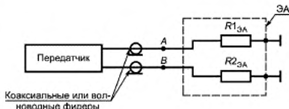
Рисунок Д.1 — Схема измерения мощности передатчика с симметричным ВЧ-выходом
