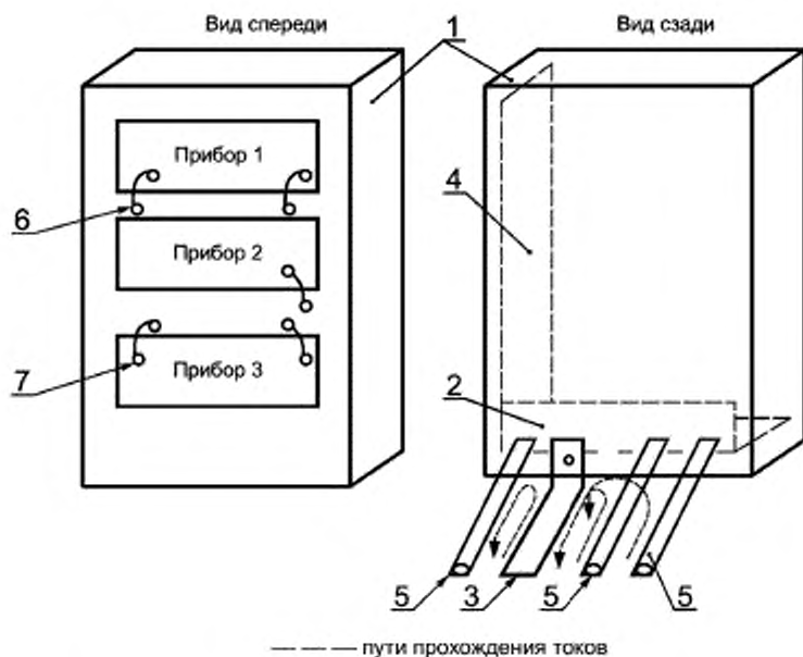
1 — экранирующий шкаф для размещения измерительных приборов; 2 — панель подключения; 3 — шина заземления шкафа; 4 — шина заземления экранирующих кожухов приборов внутри шкафа; 5 — экранированные (в двойном экране) сигнальные высокочастотные и низкочастотные кабели и экранированный кабель питания; 6 — перемычка из коаксиального кабеля; 7 — коаксиальные соединители и переходы
