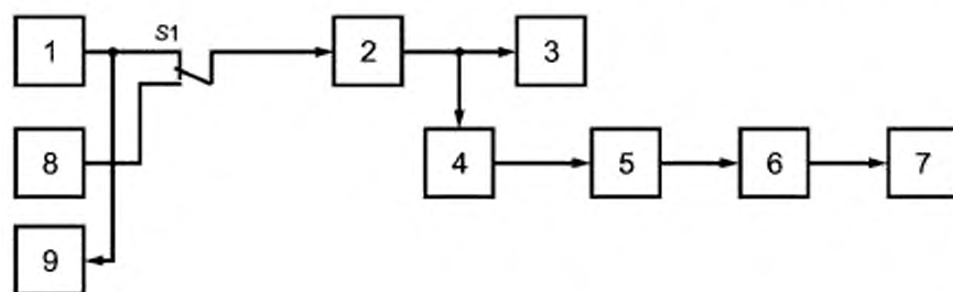
1 — генератор сигналов НЧ; 2 — передатчик; 3 — эквивалент антенны; 4 — элемент связи; 5 — анализатор модуляции (измерительный декодер); 6 — полосовой фильтр; 7 — милливольметр НЧ; 8 — экранированный резистор сопротивлением (600 \pm 30) Ом; 9 — милливольметр НЧ
