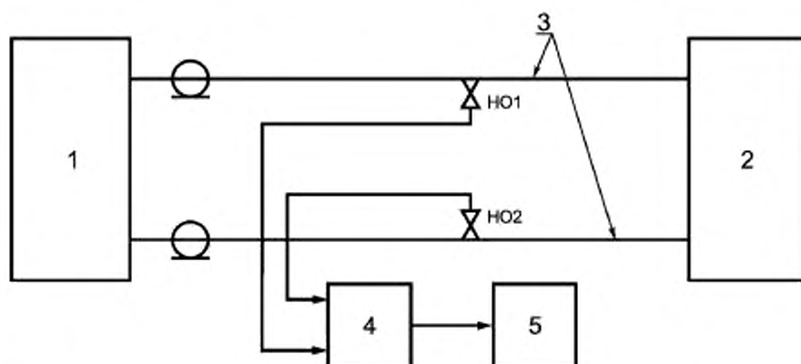
1 — передатчик; 2 — симметричная антенна или ее эквивалент; 3 — двухпроводный коаксиальный симметричный фидер; 4 — сумматор противофазных сигналов; 5 — СИ; NO1, NO2 — направленные ответвители падающих волн
