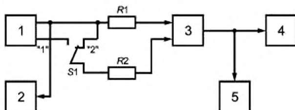
Рисунок 18 — Схема измерения коэффициента асимметрии входа телефонного канала
