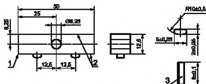
Рисунок Б.5 — Блок нагрузки с сапфирами
