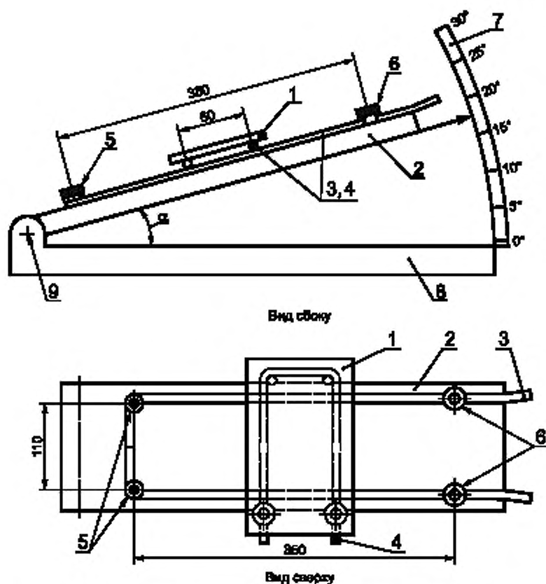
1 — блок; 2 — пластина; 3, 4 — образец провода; 5 — стойки; 6 — зажимы; 7 — шкала; 8 — основание; 9 — ось
