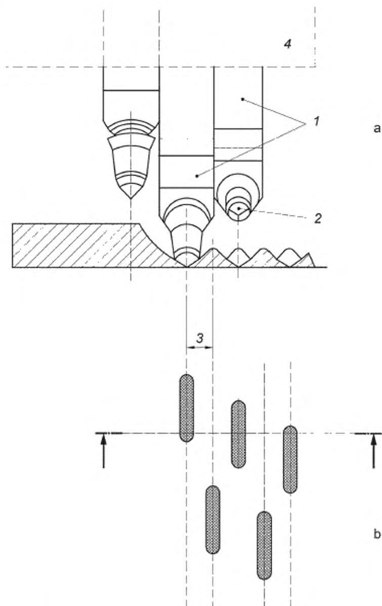
а — поперечное сечение дорожного покрытия и расположение резцов; б — вид сверху, следы от резцов; 1 — резцедержатель, 2 — режущий наконечник; 3 — шат между резцами; 4 — фрезерный барабан
